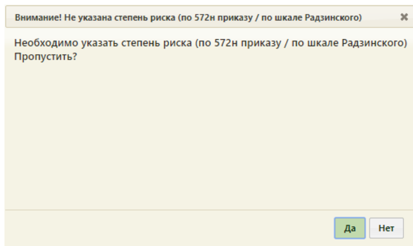
Рисунок 1268. Предупреждающее сообщение
