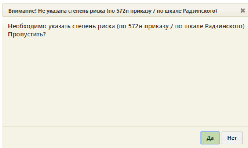
Рисунок 1122. Предупреждающее сообщение
