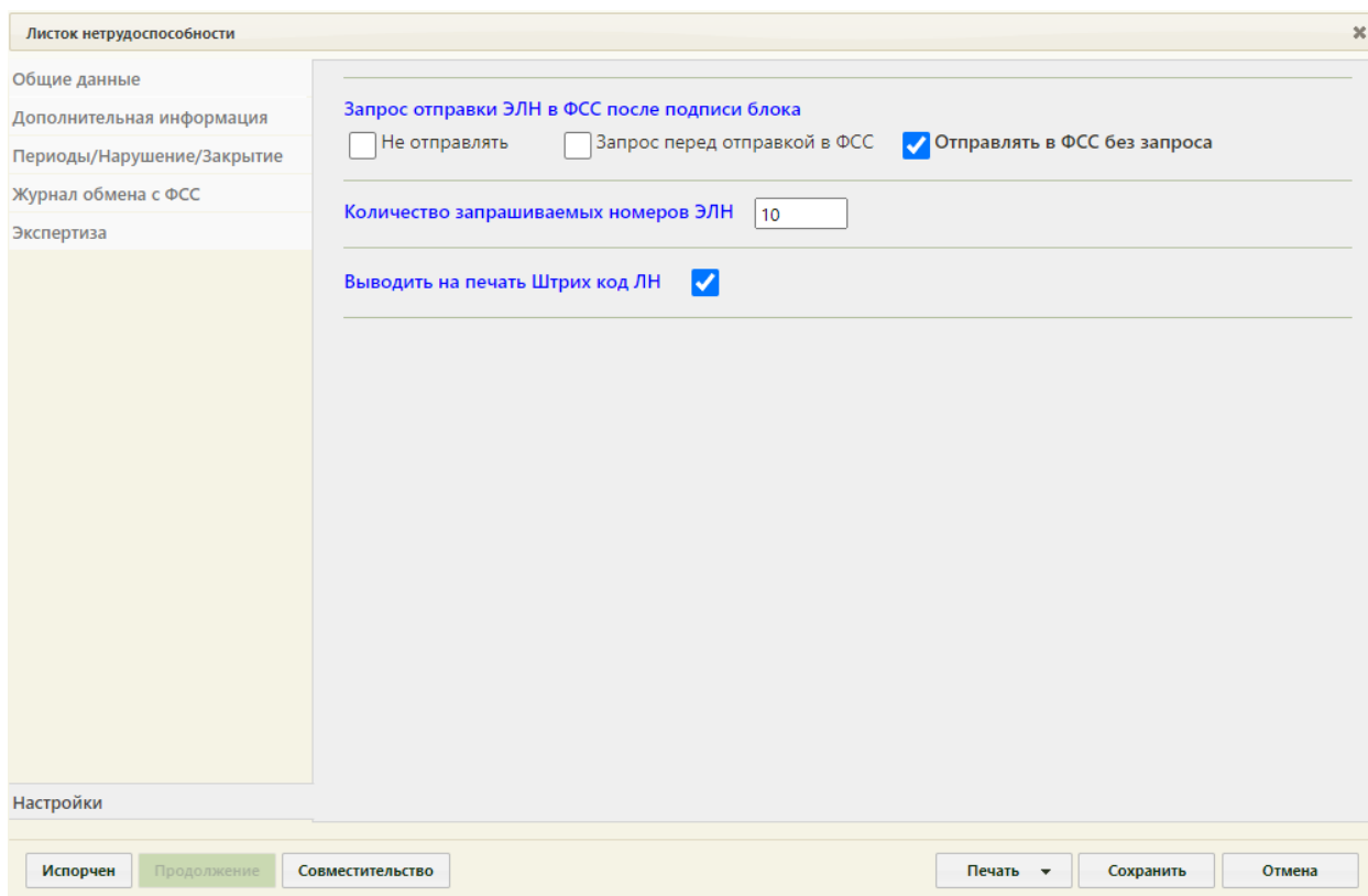
Рисунок 1437. Вкладка «Настройки»
