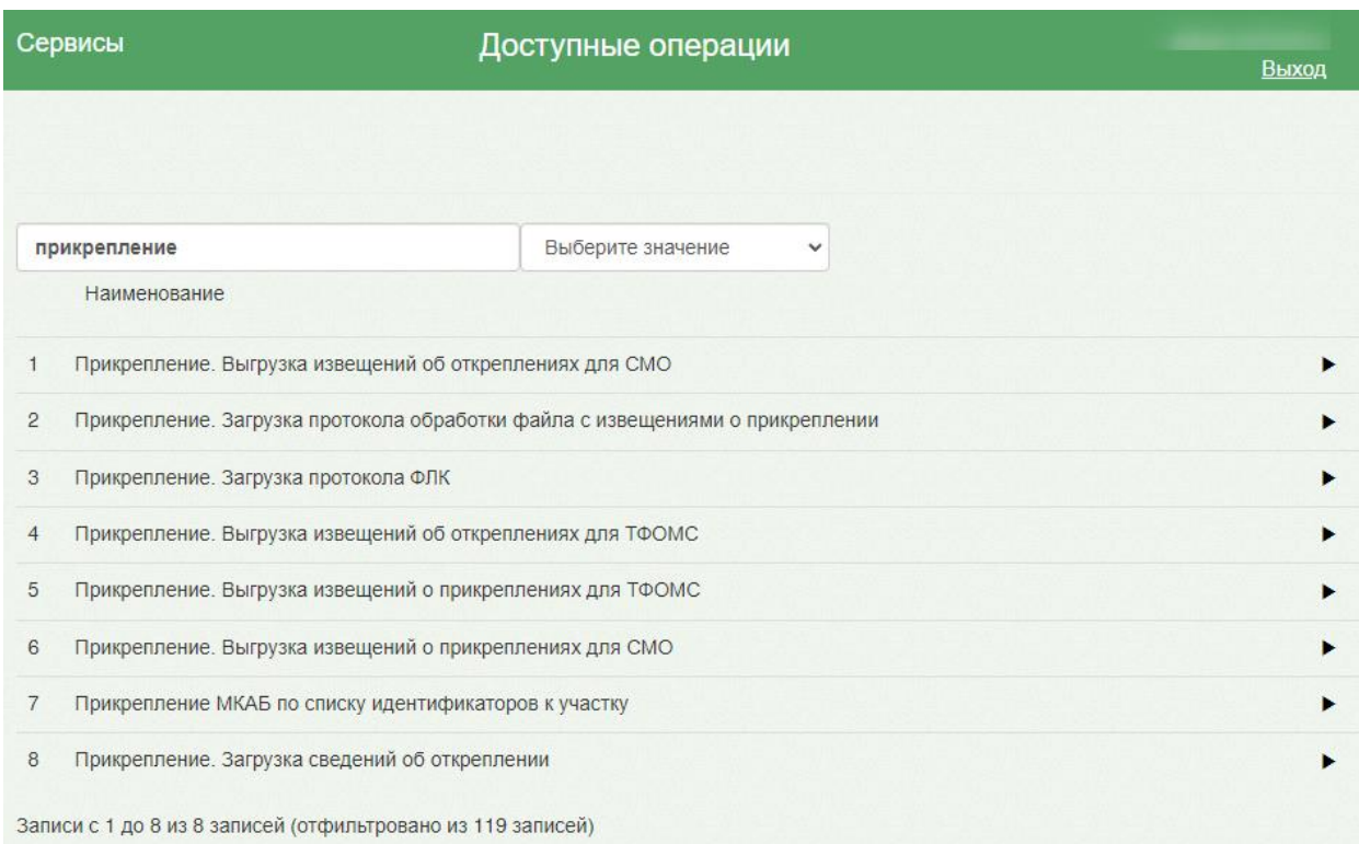
Рисунок 309. Поиск протокола
