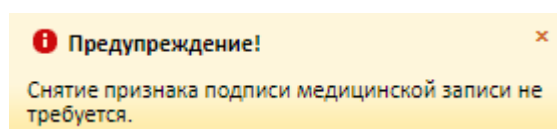
Рисунок 1196. Предупреждающее сообщение
