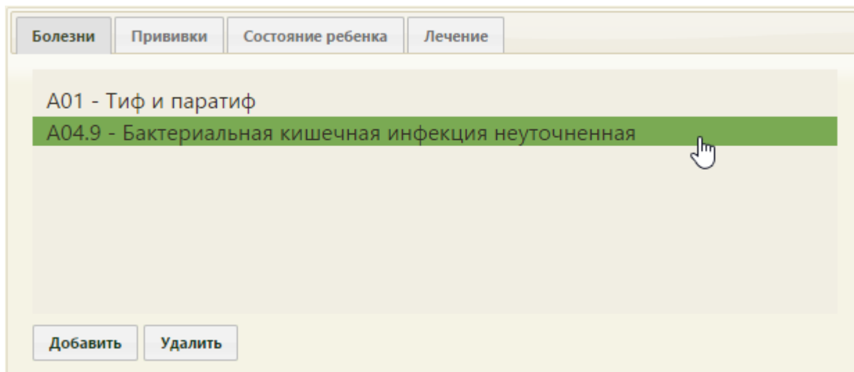
Рисунок 1217. Вкладка «Болезни»
