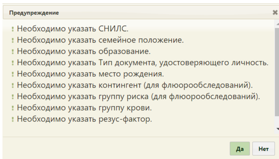
Рисунок 638. Предупреждающее сообщение
