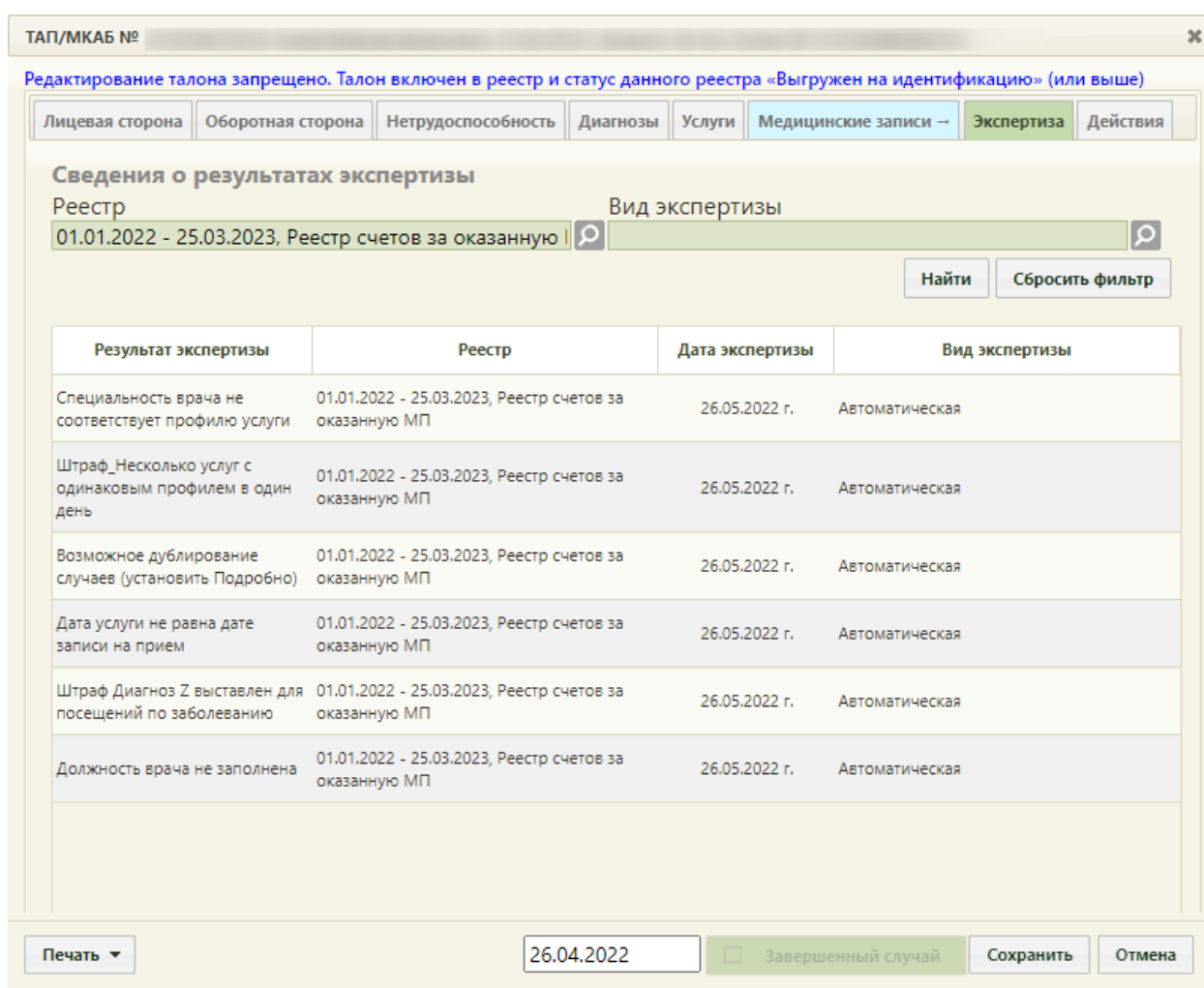
Рисунок 955. Вкладка «Экспертиза»
