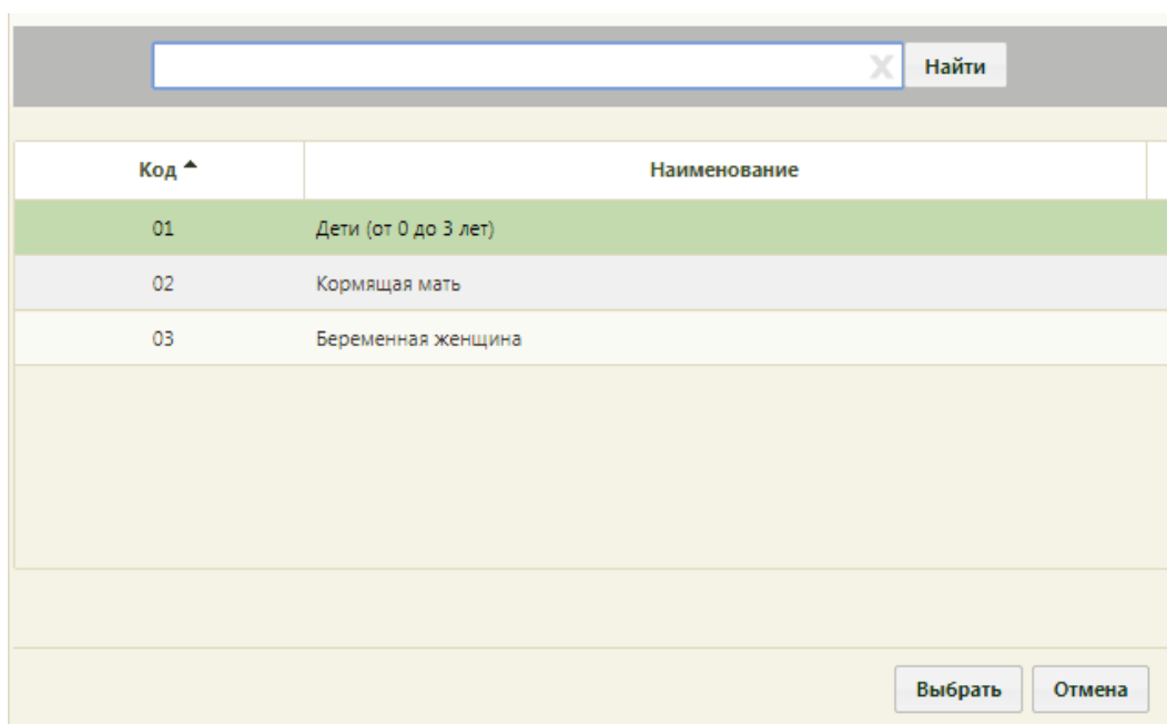
Рисунок 1690. Справочник «Категория»
