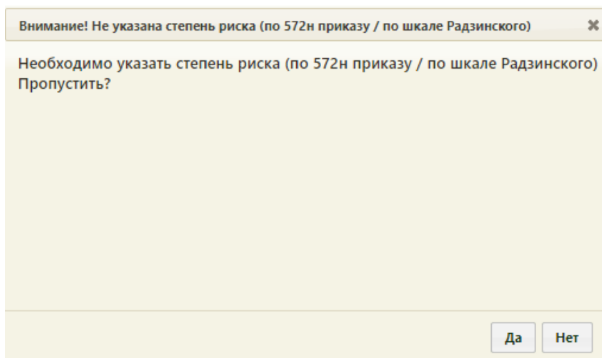
Рисунок 1167. Предупреждающее сообщение
