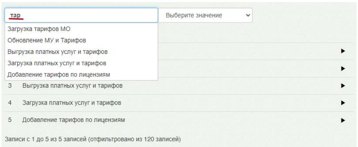
Рисунок 1610. Поиск протокола
