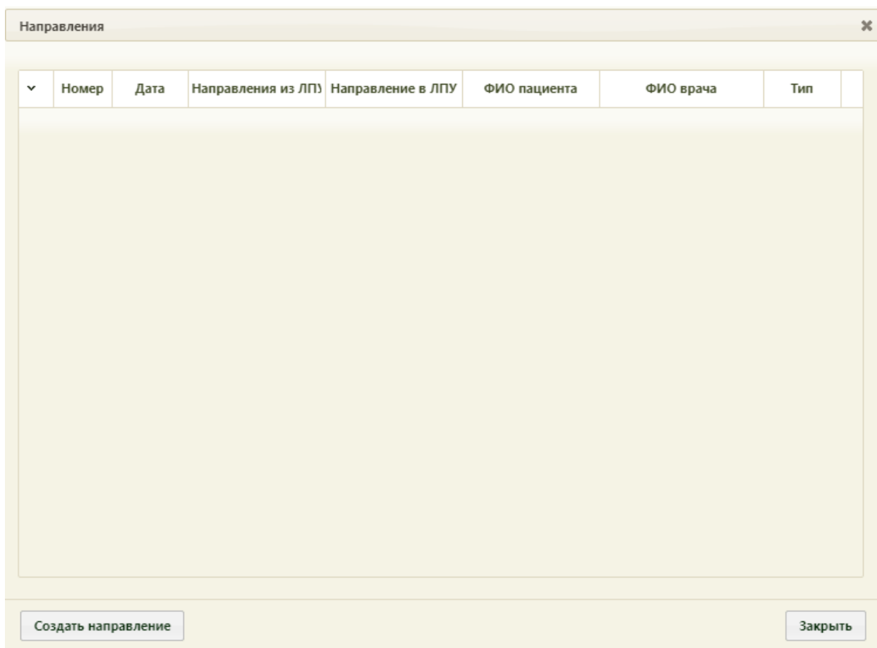
Рисунок 965. Форма «Направления»
