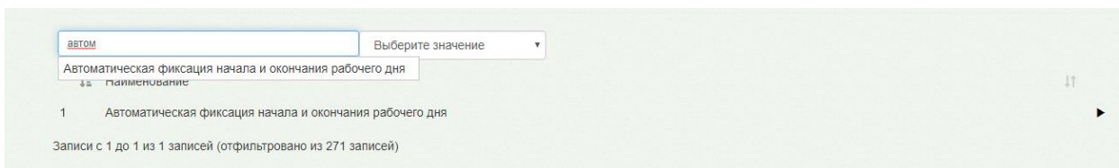
Рисунок 1934. Поиск отчета
