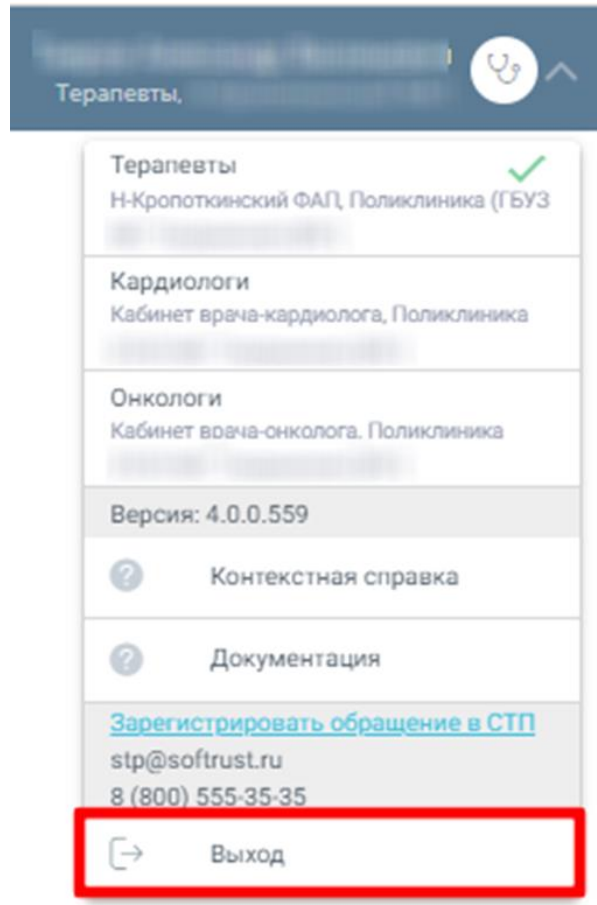
Рисунок 864. Закрытие журнала
