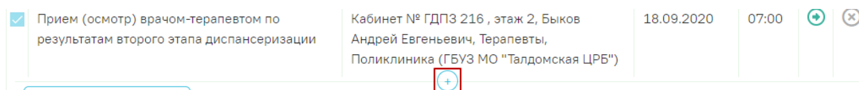
Рисунок 657. Кнопка «Добавить»
