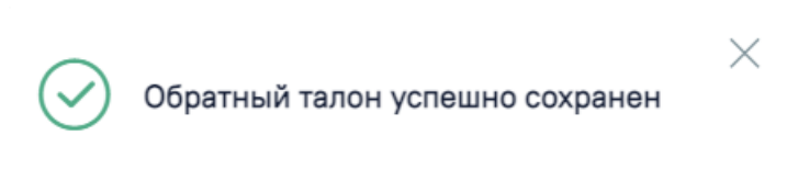
Рисунок 2085. Информационное сообщение
