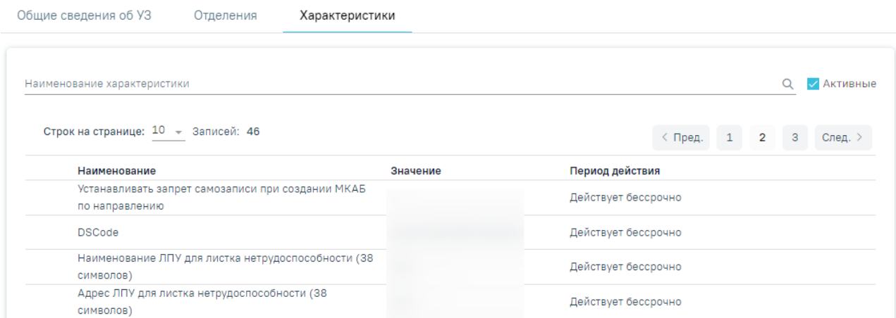
Рисунок 2895. Вкладка «Характеристики»
