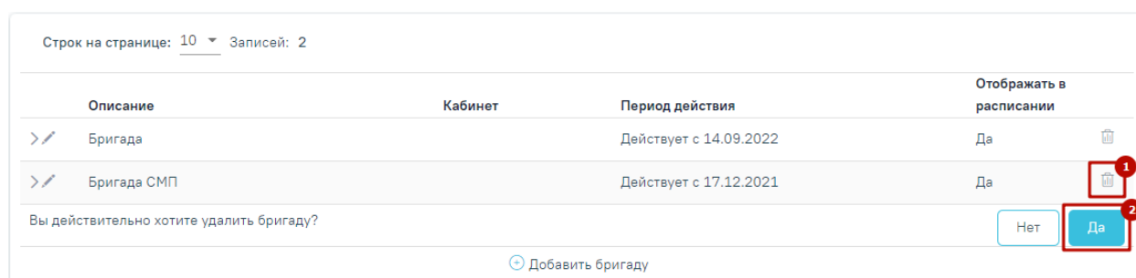
Рисунок 2976. Удаление бригады
