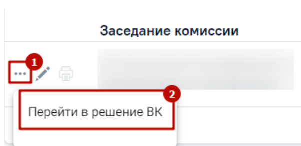
Рисунок 488. Дополнительные действия
