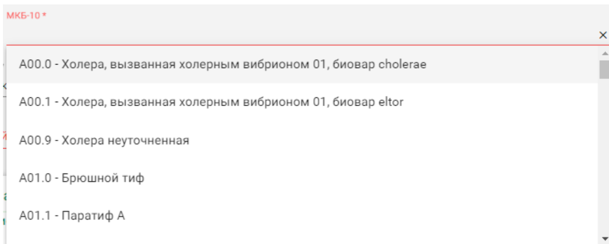
Рисунок 340. Список диагнозов
