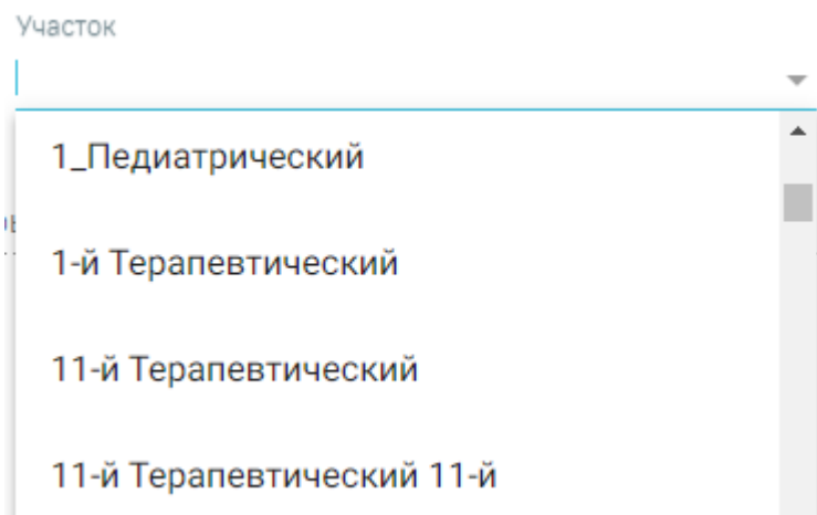
Рисунок 2604. Список участков
