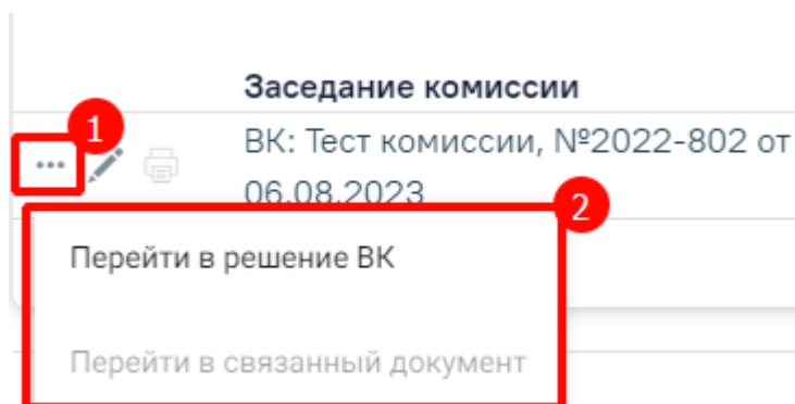
Рисунок 2115. Дополнительные действия
