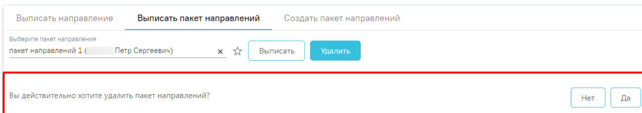
Рисунок 229. Подтверждение действия
