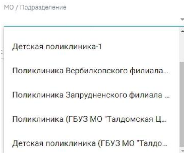
Рисунок 2603. Выбор МО/подразделения
