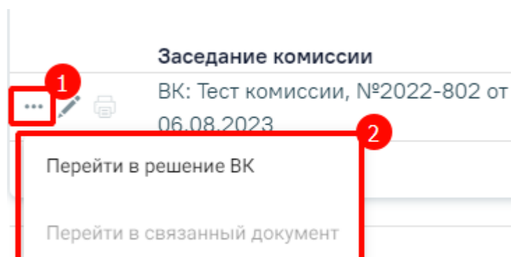
Рисунок 2119. Дополнительные действия
