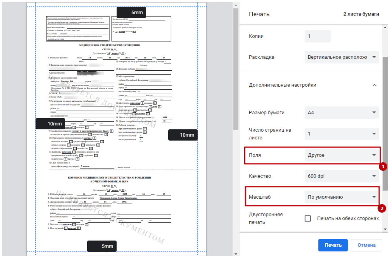
Рисунок 1132. Настройка печати
