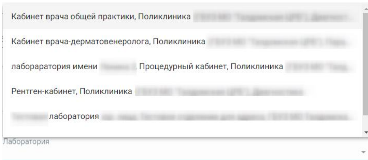
Рисунок 347. Выбор лаборатории
