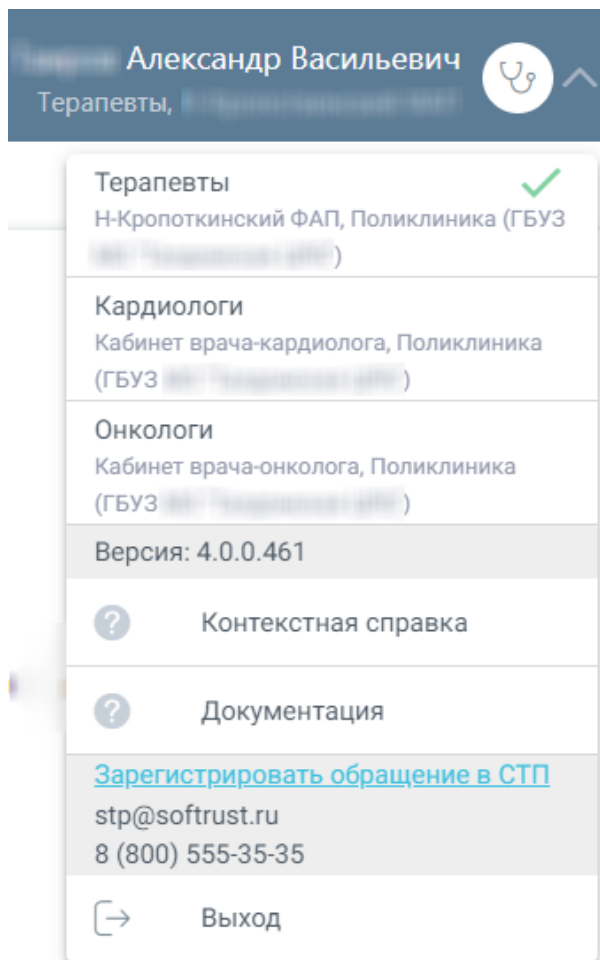
Рисунок 933. Пункты меню
