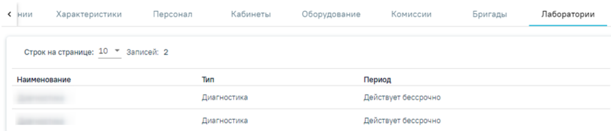
Рисунок 2897. Вкладка «Лаборатории»
