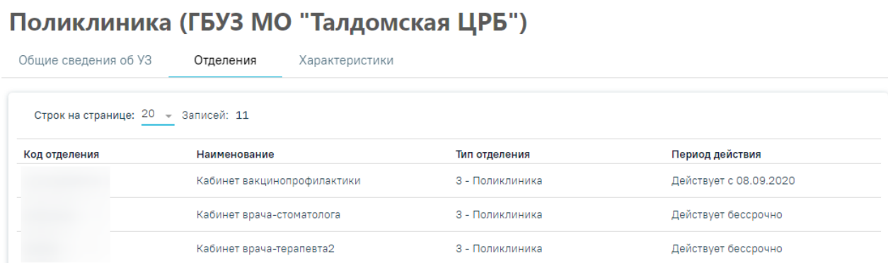
Рисунок 2893. Вкладка «Отделения»
