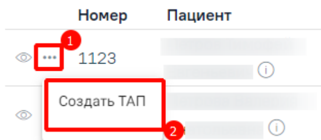
Рисунок 2623. Создание ТАП
