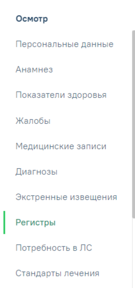
Рисунок 1586. Вкладка «Регистры»
