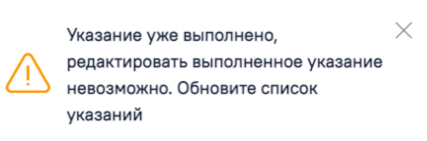
Рисунок 1727. Предупреждающее сообщение
