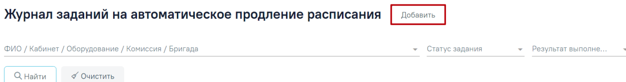
Рисунок 2782. Кнопка «Добавить»
