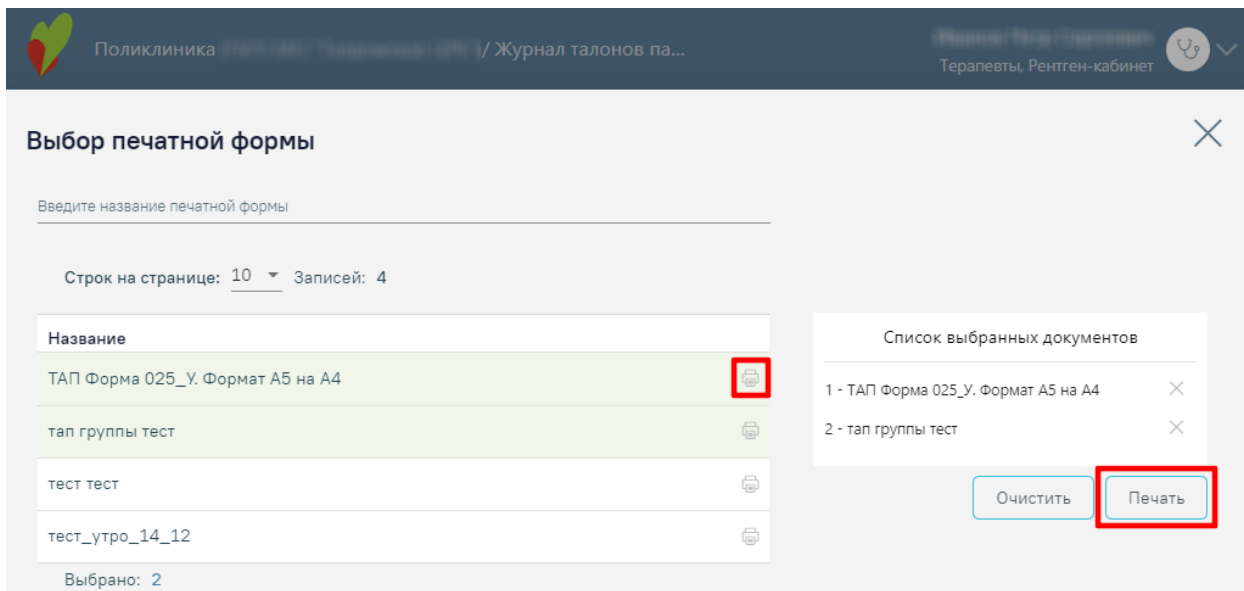
Рисунок 3140. Раздел «Отчеты»
