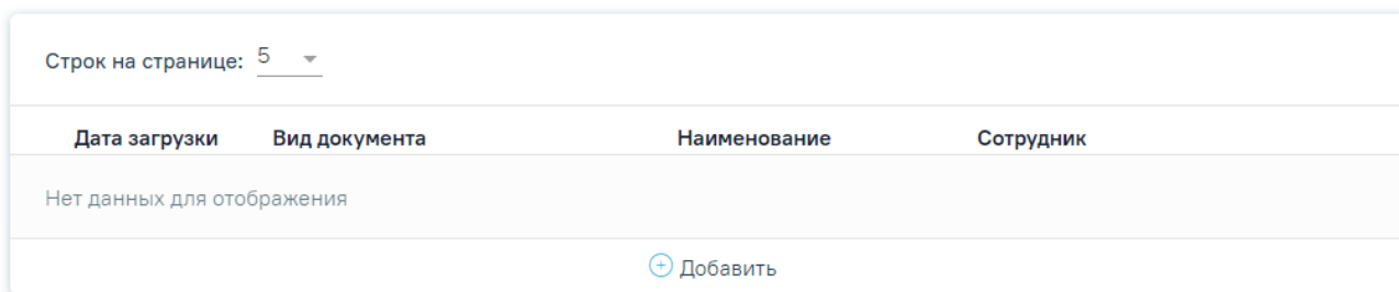
Рисунок 2705. Блок «Документы»
