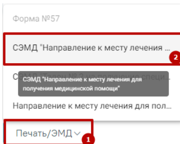
Рисунок 504. Кнопка «Печать/ЭМД»
