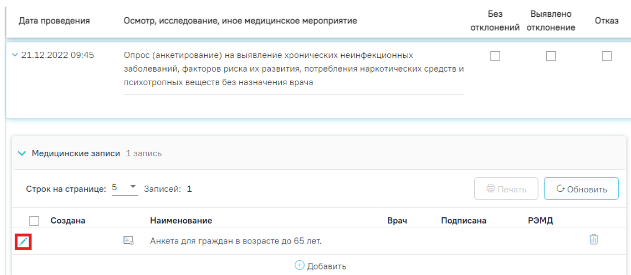
Рисунок 810. Кнопка «Редактировать»
