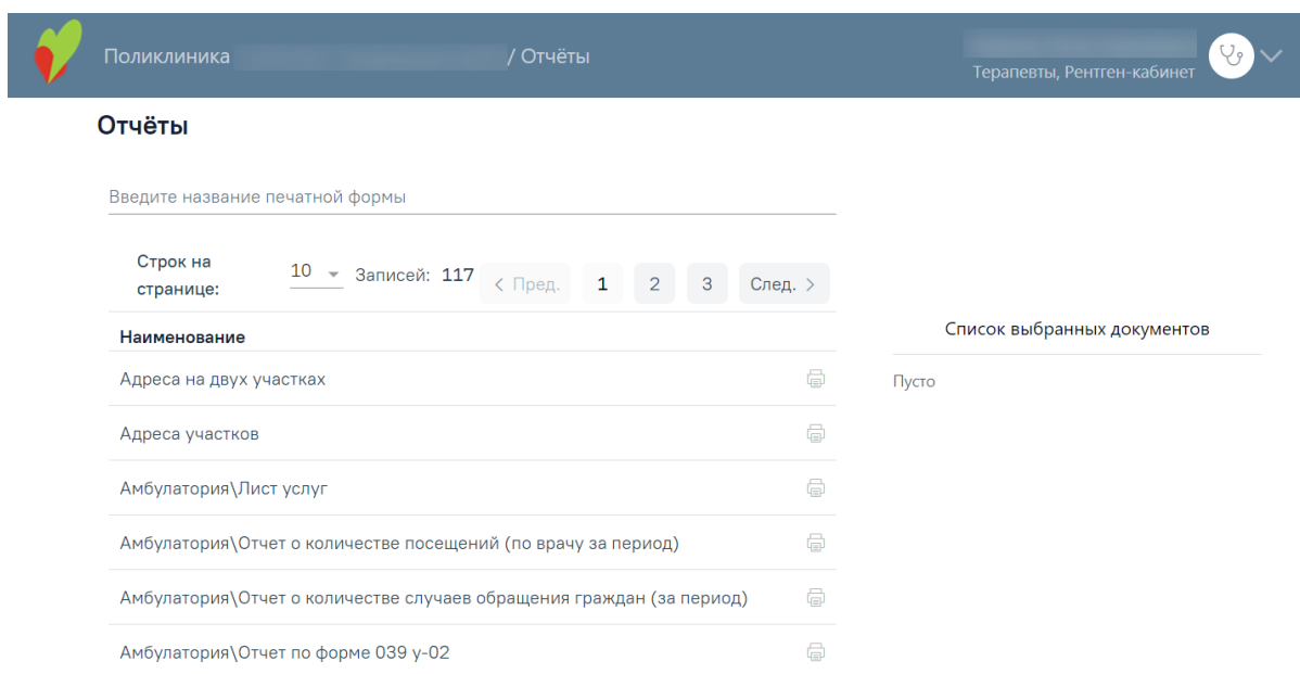
Рисунок 3142. «Отчёты»
