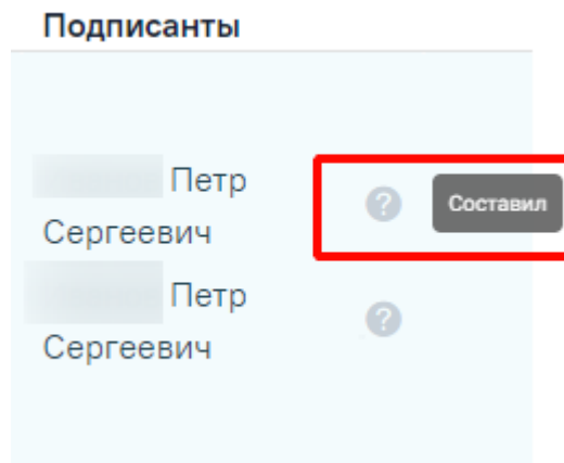
Рисунок 2752. Роль подписанта
