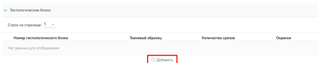
Рисунок 1364. Кнопка «Добавить»
