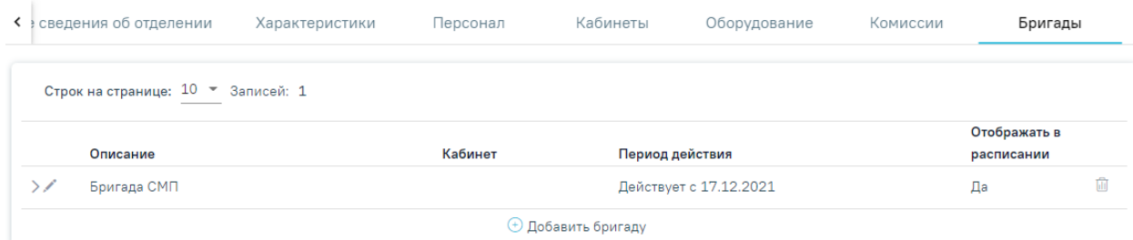
Рисунок 2965. Вкладка «Бригады»
