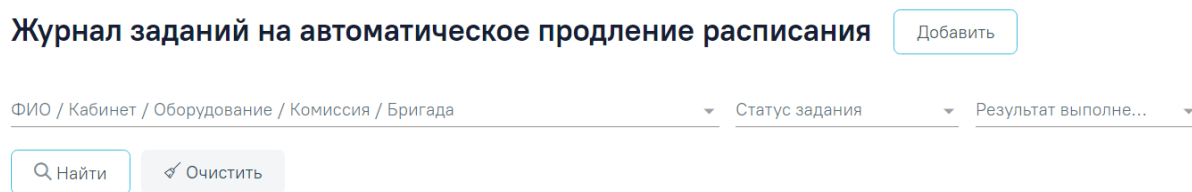
Рисунок 2776. Панель фильтрации
