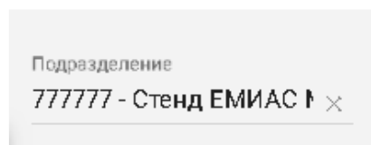
Рисунок 935. Установление подразделения
