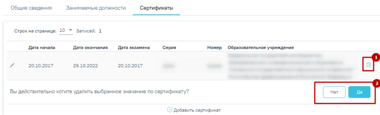
Рисунок 3005. Удаления сертификата
