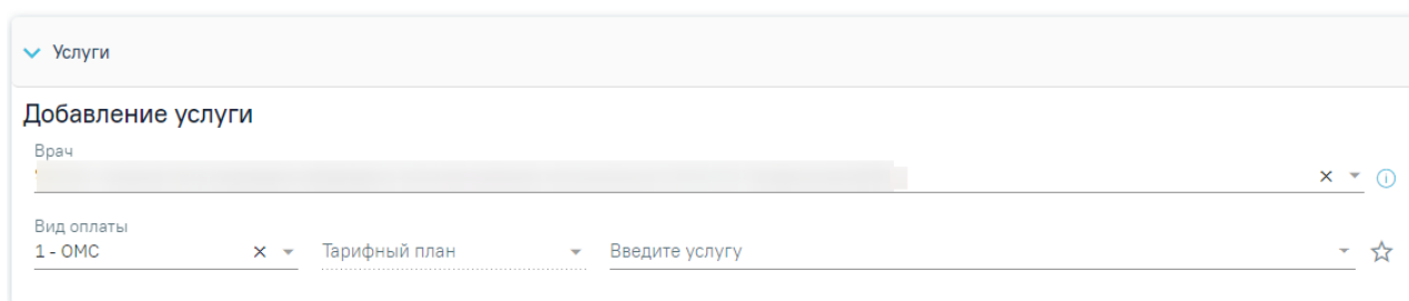
Рисунок 301. Блок «Услуги»
