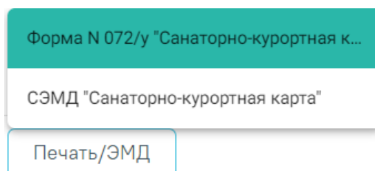
Рисунок 2086. Кнопка «Печать/ЭМД»
