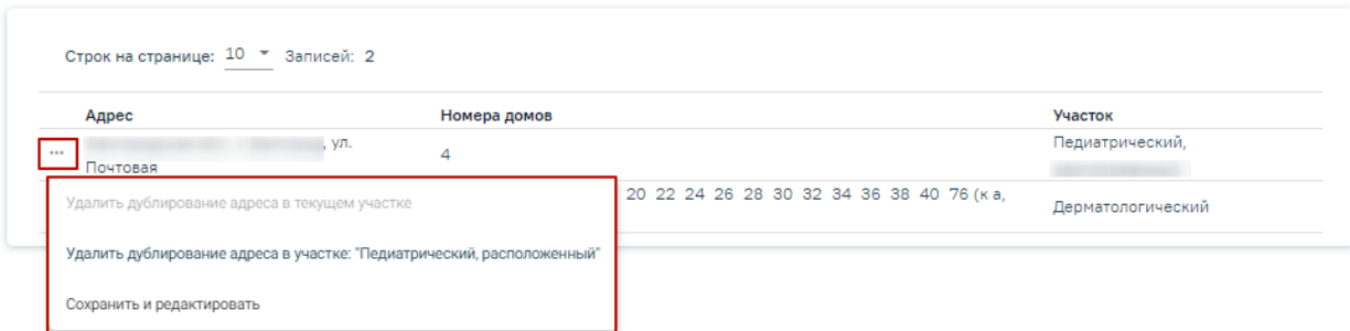
Рисунок 2815. Контекстное меню
