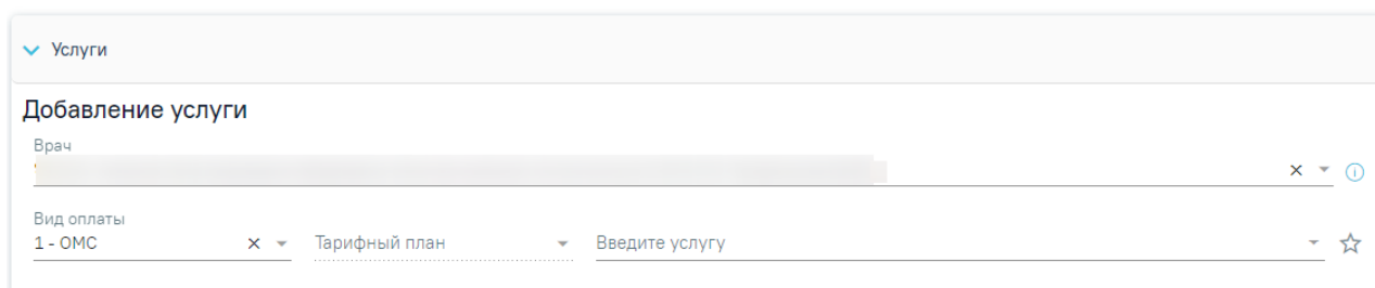
Рисунок 409. Блок «Услуги»
