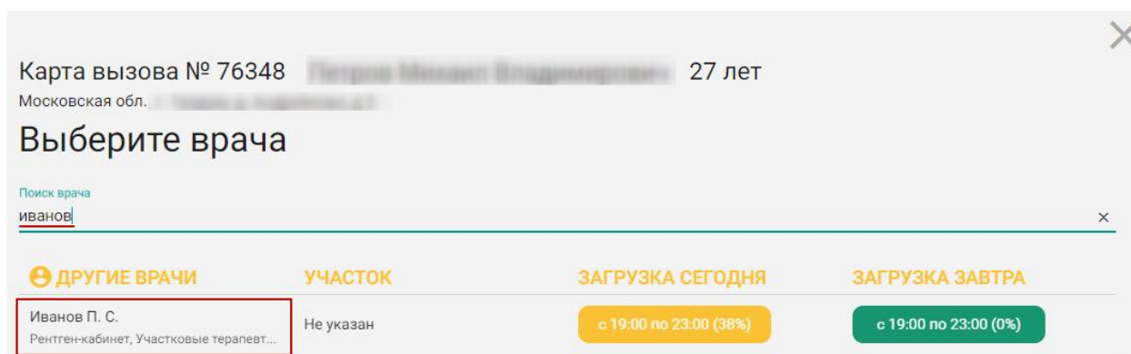
Рисунок 988. Поиск врача
