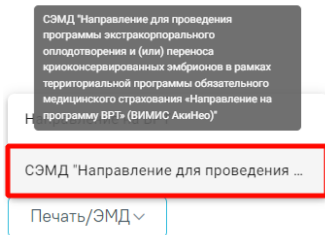
Рисунок 632. Кнопка «Печать/ЭМД»
