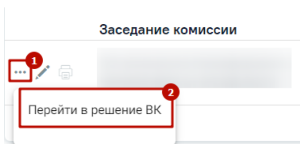
Рисунок 563. Дополнительные действия
