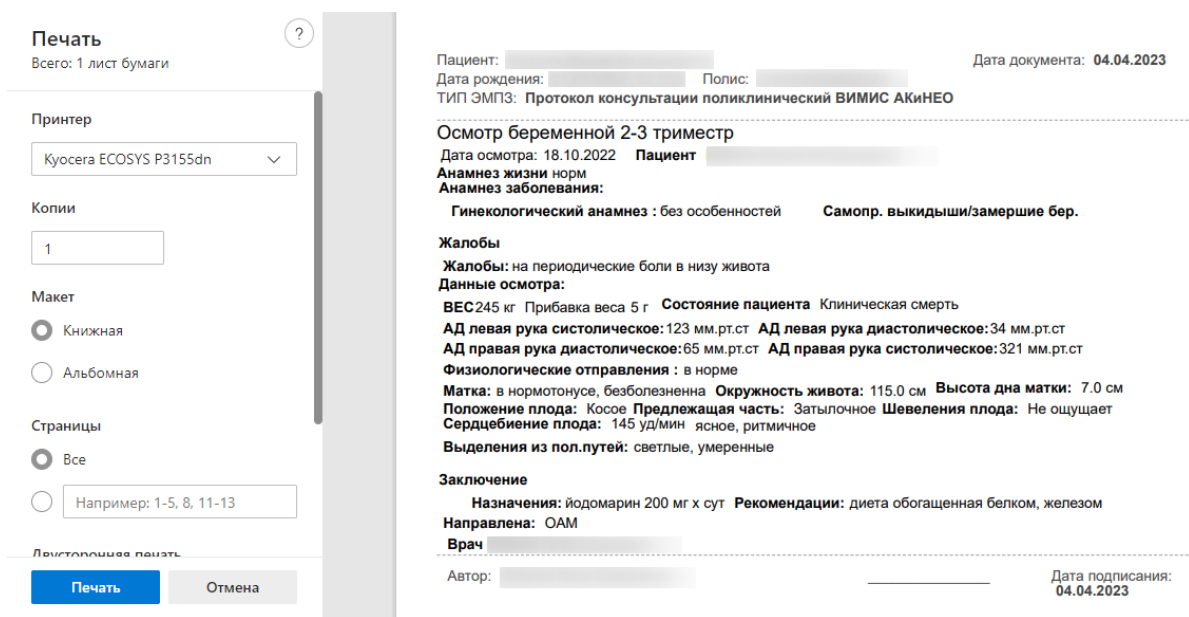
Рисунок 3093. Печать МЗ
