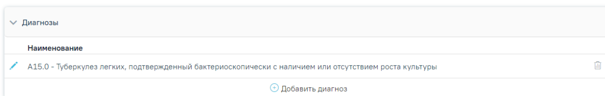
Рисунок 2213. Блок «Диагнозы»
