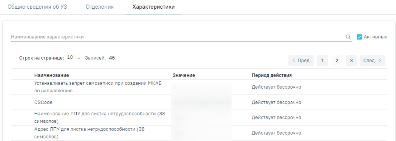
Рисунок 2081. Вкладка «Характеристики»
