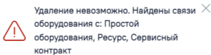
Рисунок 2131. Предупреждающее сообщение
