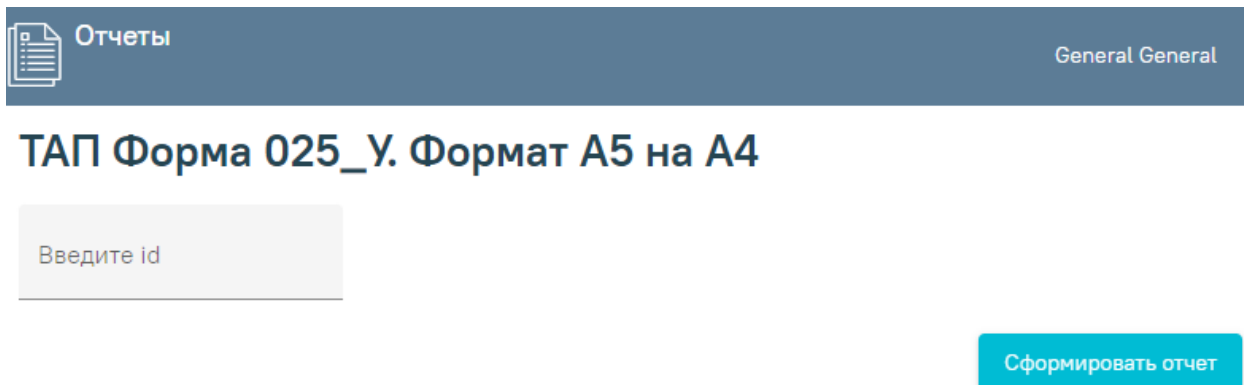
Рисунок 2374. Формирование отчета
