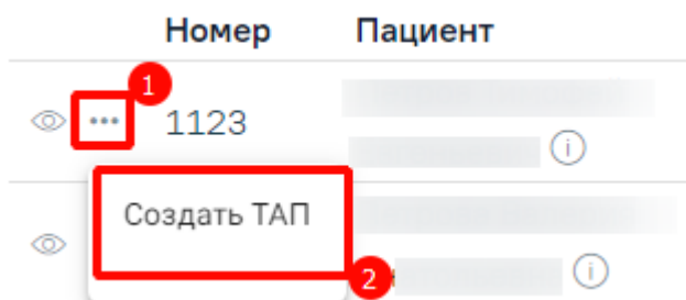
Рисунок 1777. Создание ТАП
