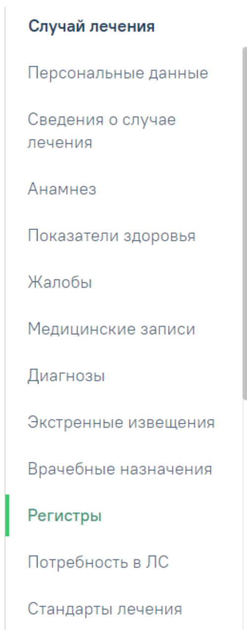
Рисунок 721. Вкладка «Регистры»
