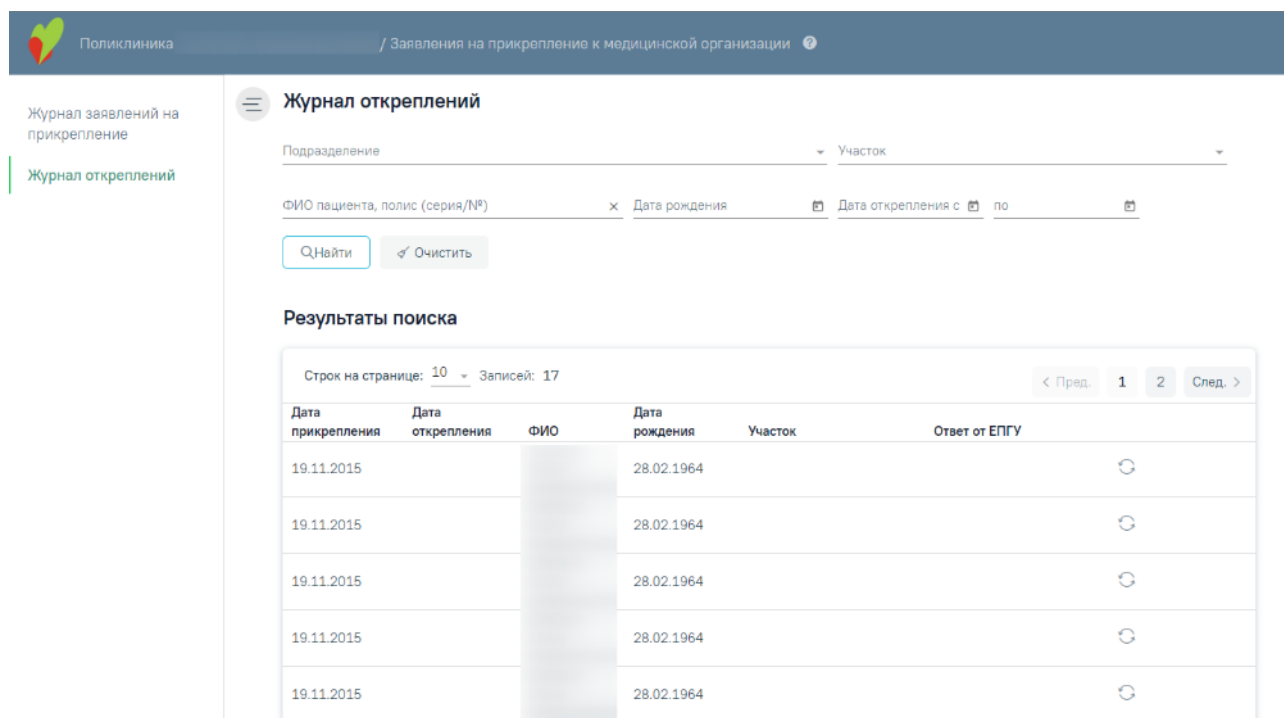
Рисунок 2102. Журнал откреплений
