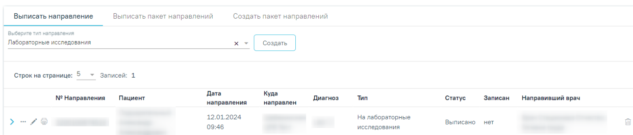
Рисунок 671. Блок «Направления»
