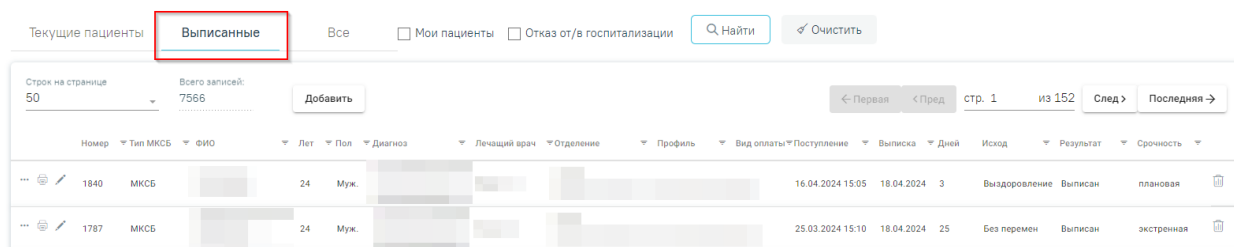
Рисунок 301. Вкладка «Выписанные»
