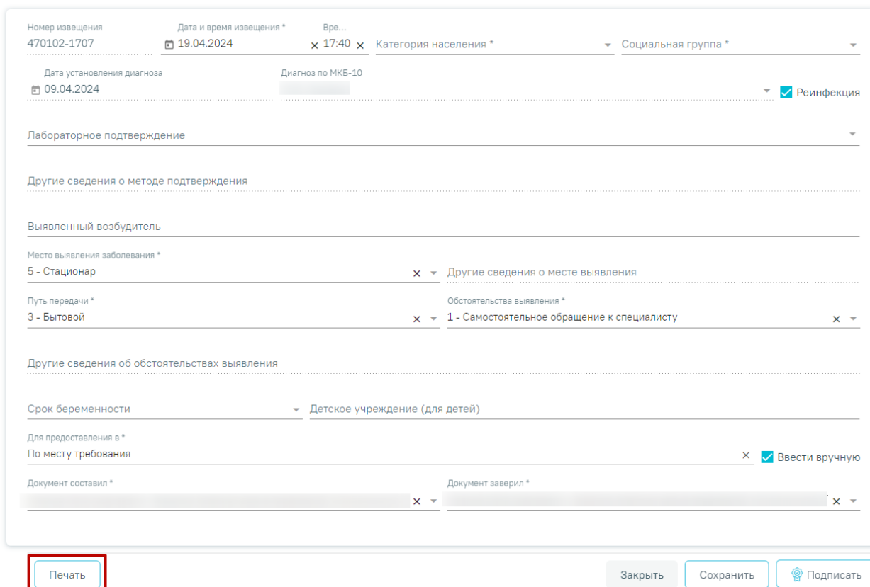
Рисунок 504. Кнопка «Печать»
