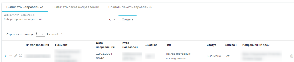
Рисунок 693. Блок «Направления»
