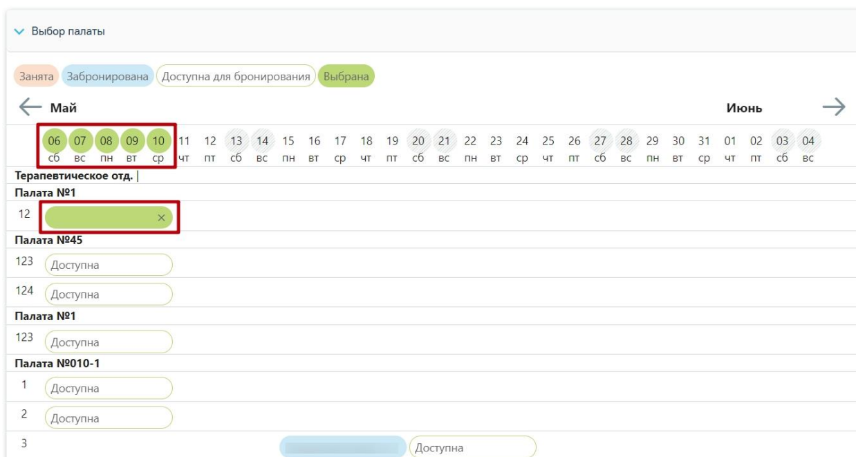
Рисунок 1029. Выбор койки
