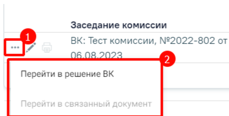
Рисунок 808. Дополнительные действия
