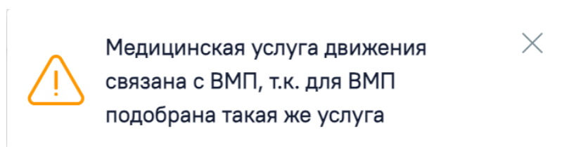
Рисунок 838. Предупреждающее сообщение
