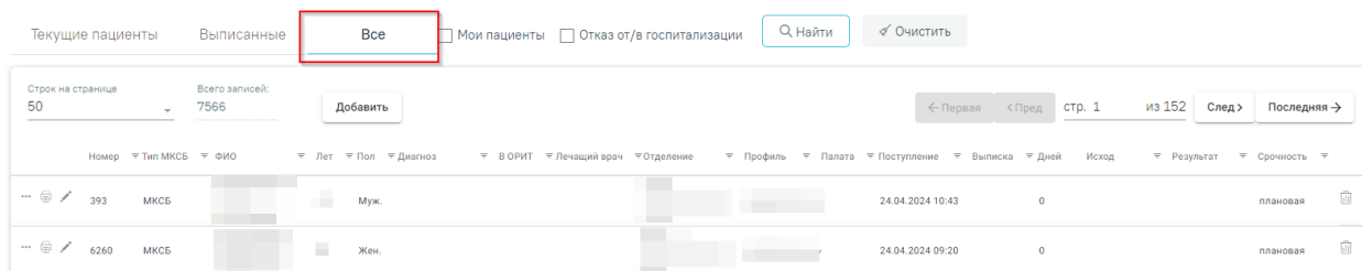
Рисунок 955. Вкладка «Все»
