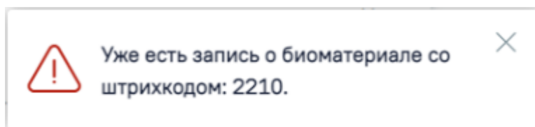
Рисунок 1640. Предупреждающее сообщение
