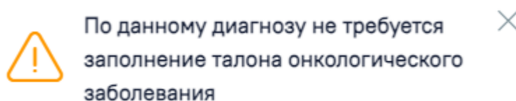
Рисунок 334. Предупреждающее сообщение
