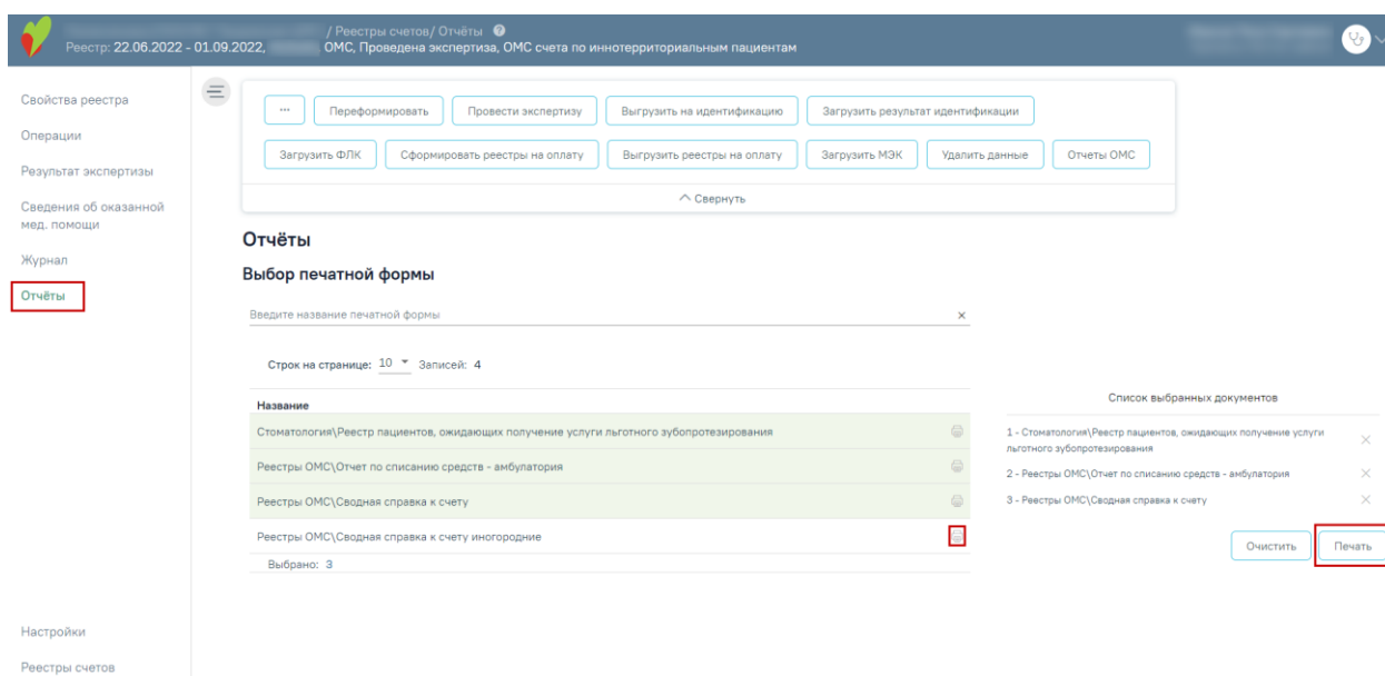
Рисунок 548. Раздел «Отчеты»
