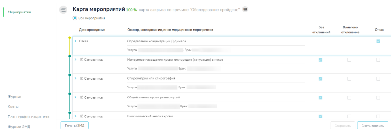
Рисунок 525. Карта мероприятий
