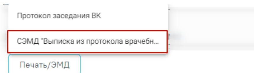
Рисунок 663. Кнопка «Печать/ЭМД»
