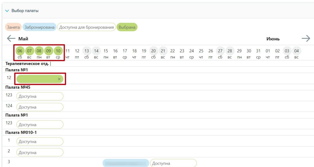
Рисунок 344. Выбор койки
