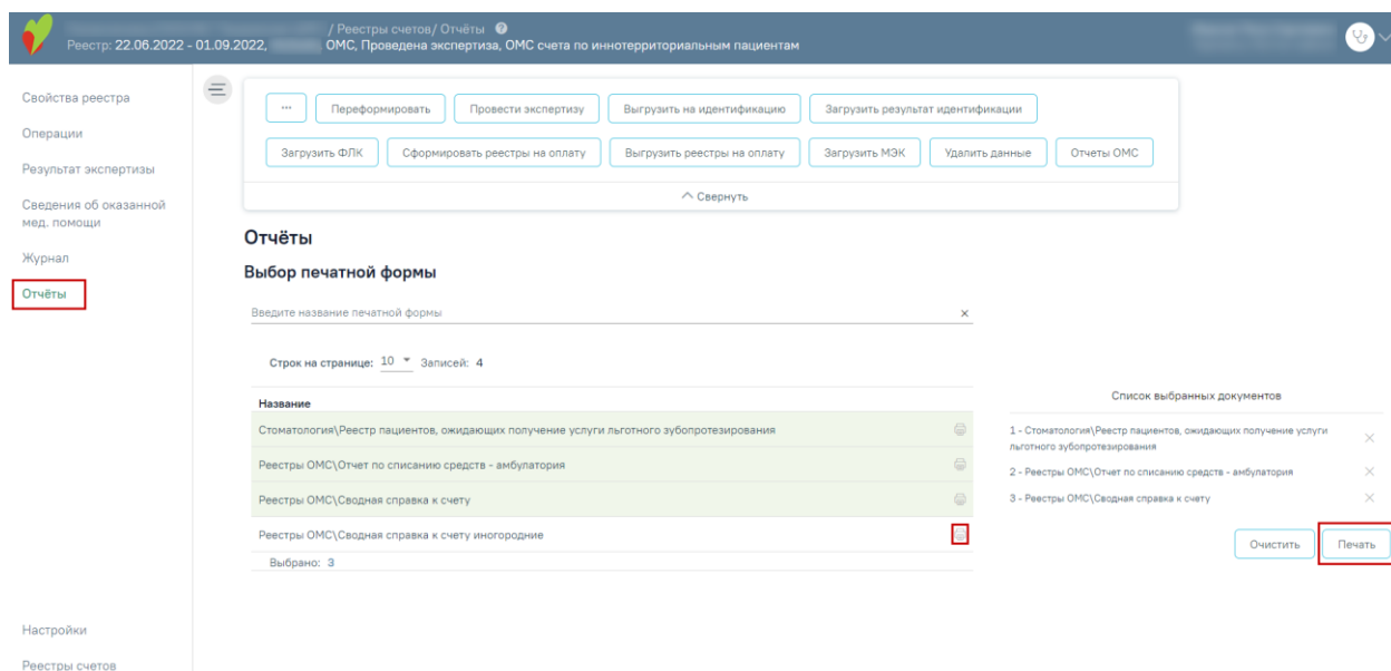
Рисунок 606. Раздел «Отчеты»
