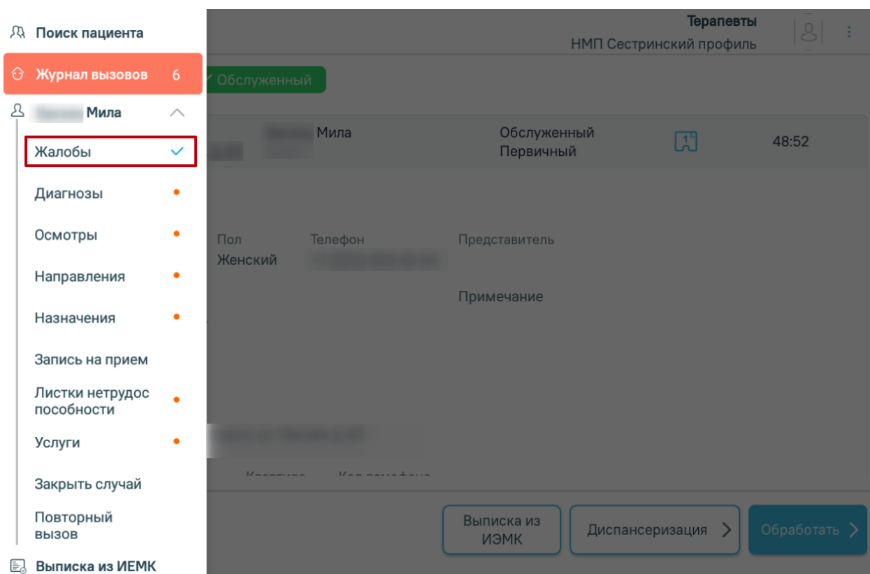
Рисунок 756. Пункт «Жалобы»
