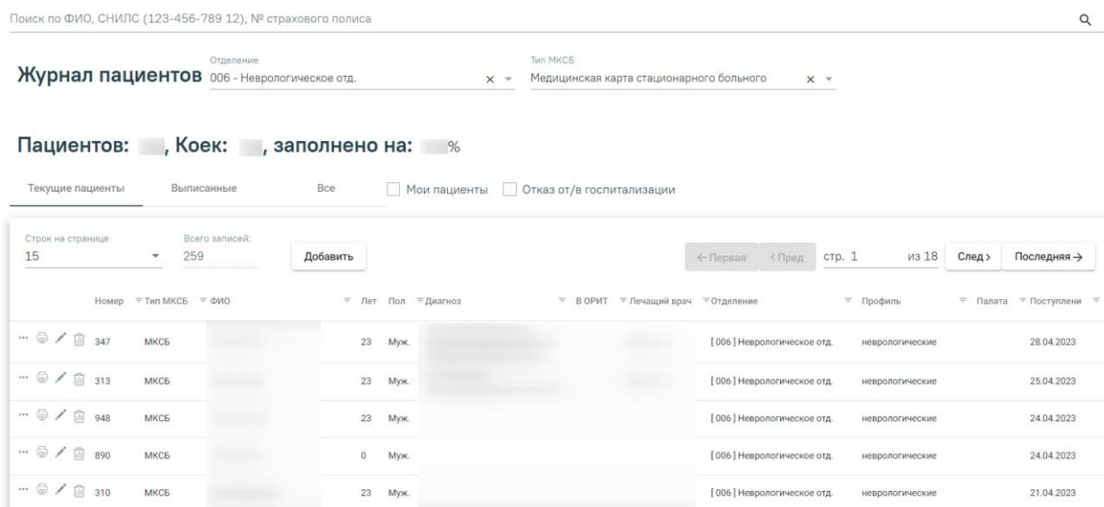
Рисунок 123. Журнал пациентов
