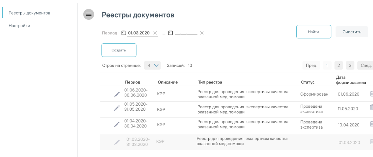
Рисунок 740. Реестры документов
