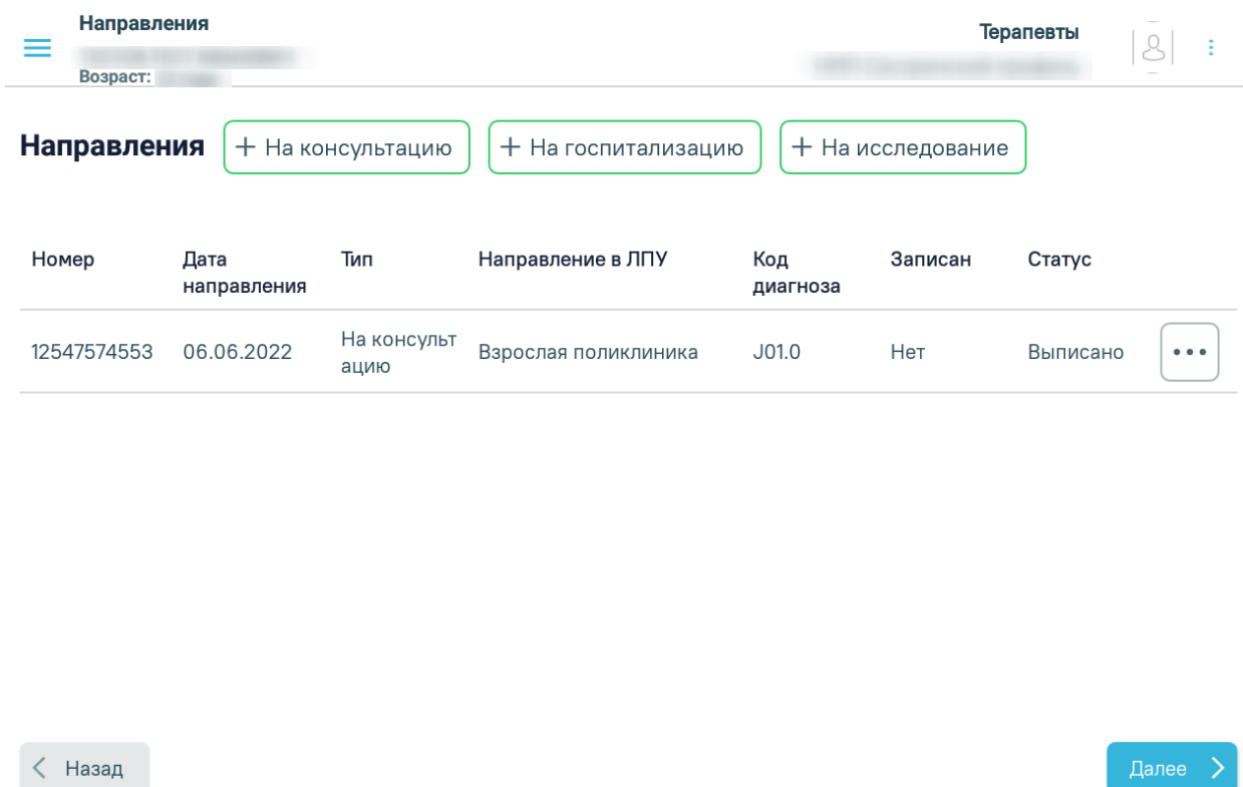
Рисунок 784. Форма «Направления»
