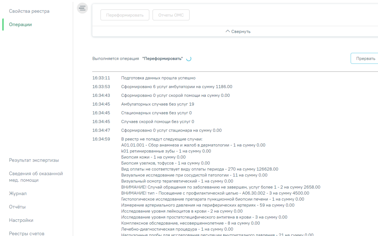
Рисунок 564. Раздел «Операции»
