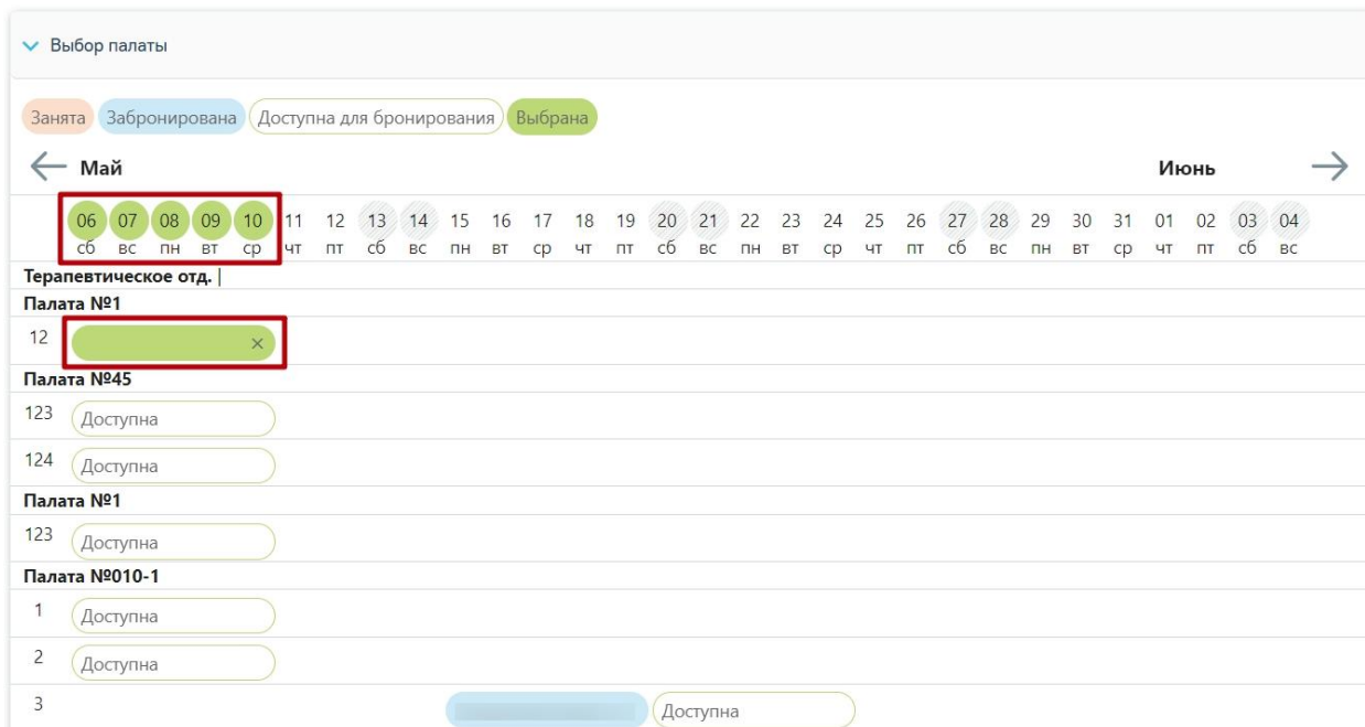
Рисунок 400. Выбор койки
