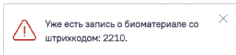
Рисунок 851. Предупреждающее сообщение
