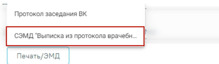
Рисунок 730. Кнопка «Печать/ЭМД»
