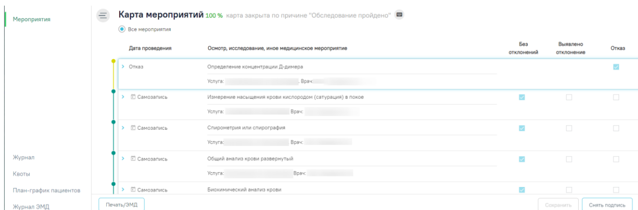
Рисунок 583. Карта мероприятий
