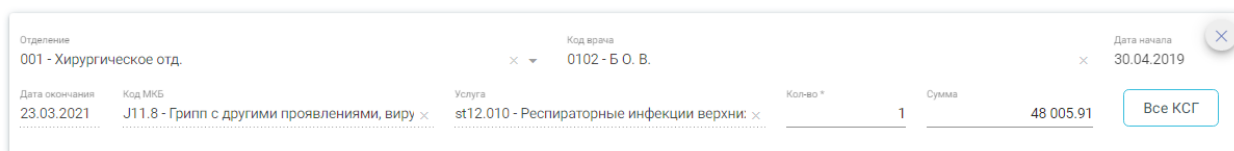
Рисунок 234. Блок «КСГ»
