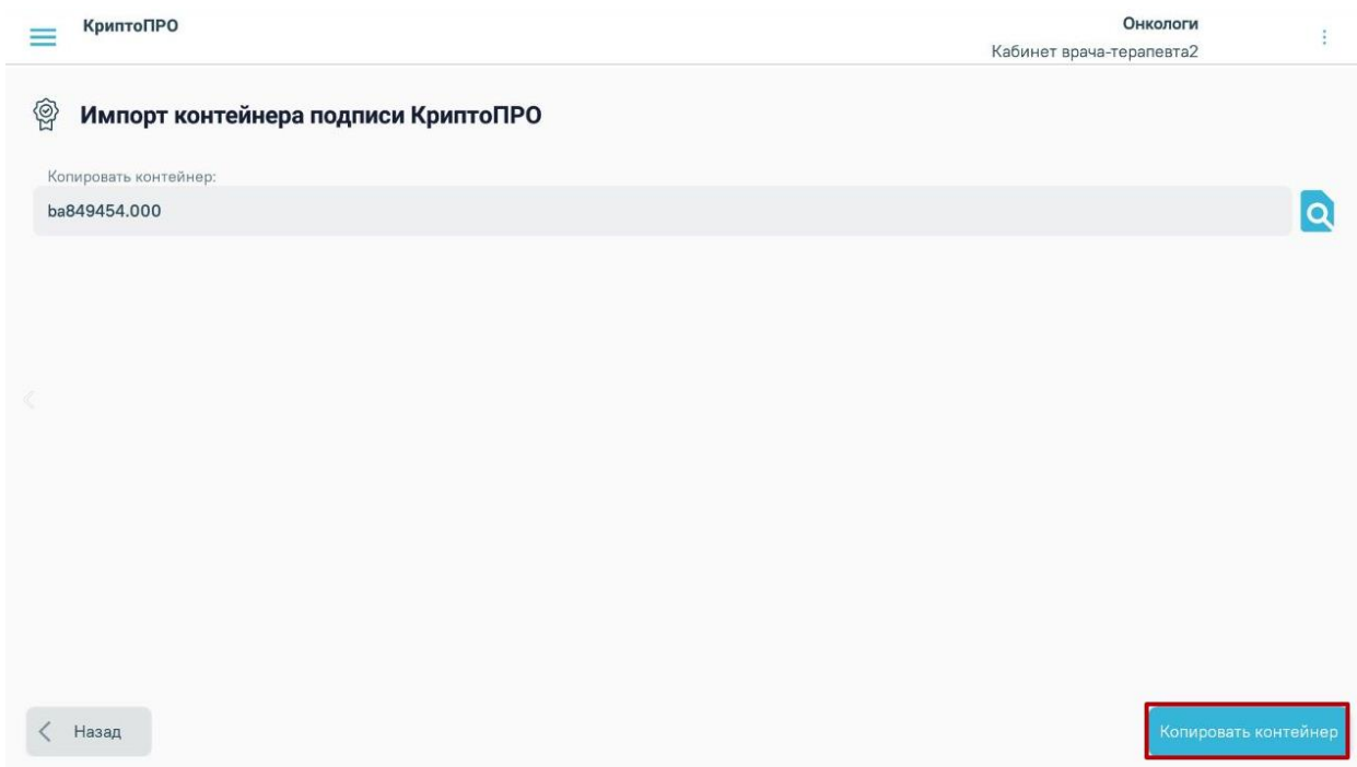
Рисунок 881. Выбор контейнера
