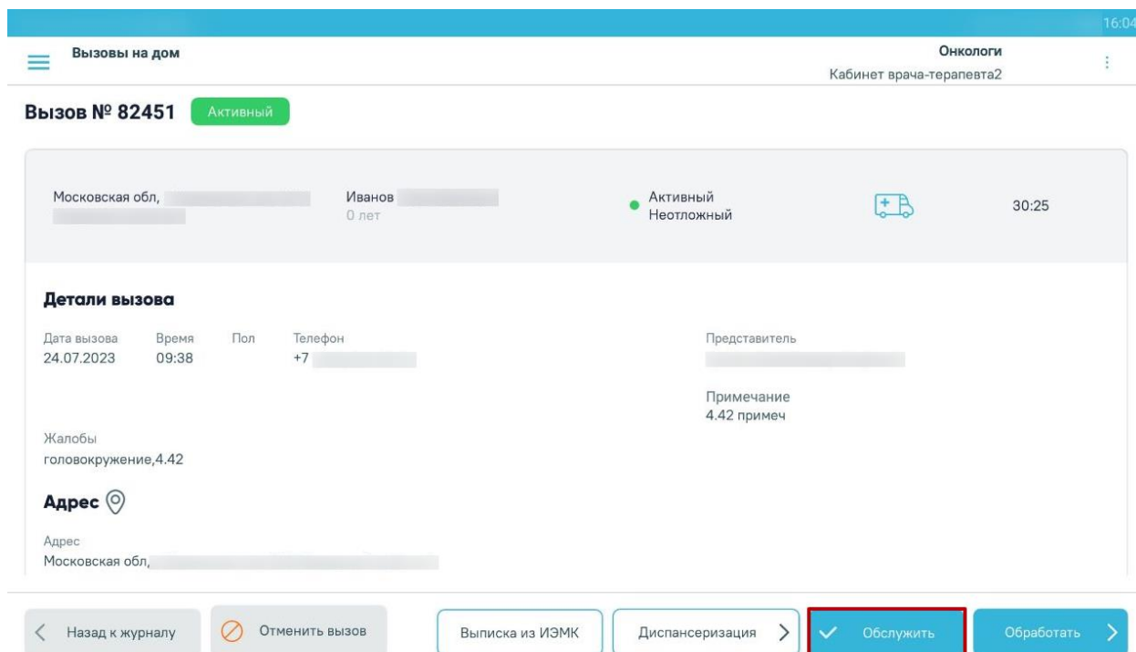
Рисунок 775. Кнопка «Обслужить»
