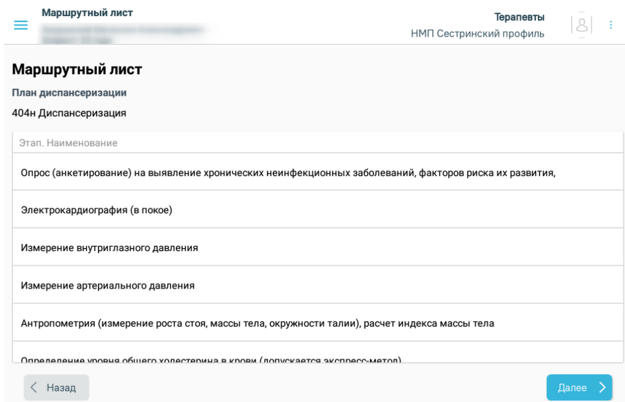
Рисунок 862. План диспансеризации
