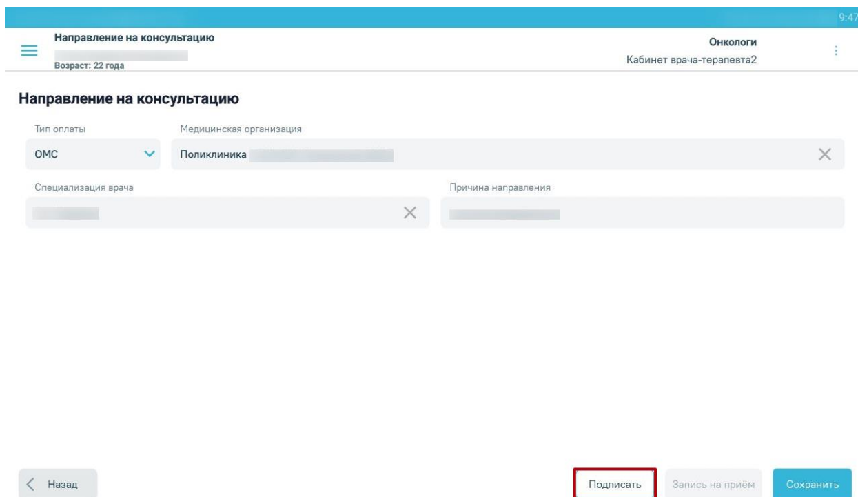
Рисунок 804. Кнопка «Подписать»
