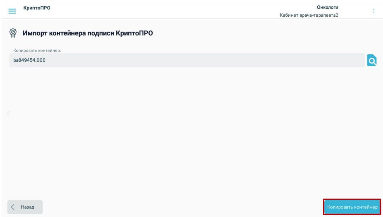
Рисунок 1334. Выбор контейнера
