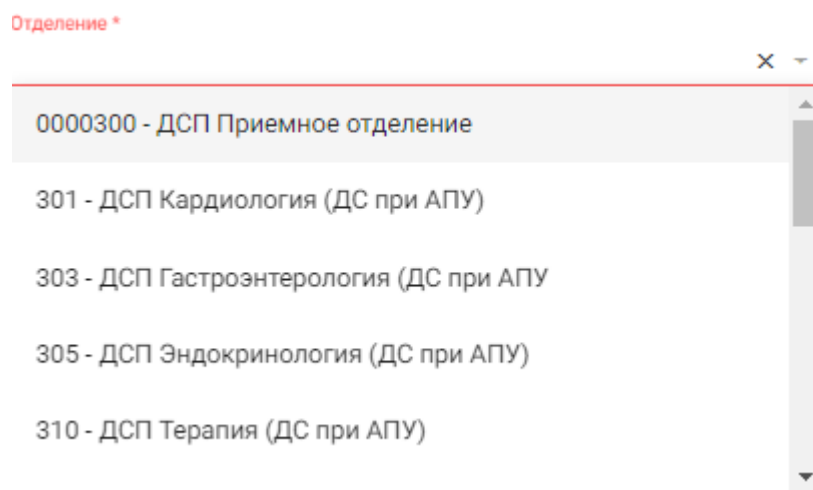
Рисунок 789. Поле «Отделение»
