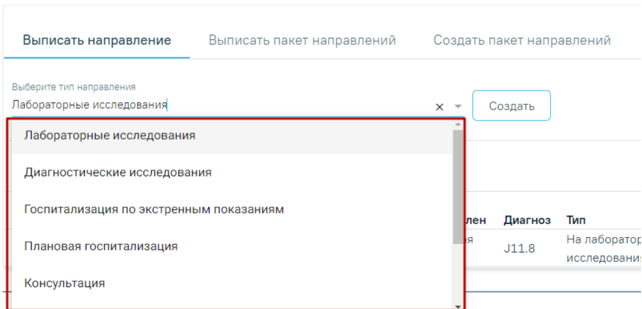
Рисунок 574. Создание направления
