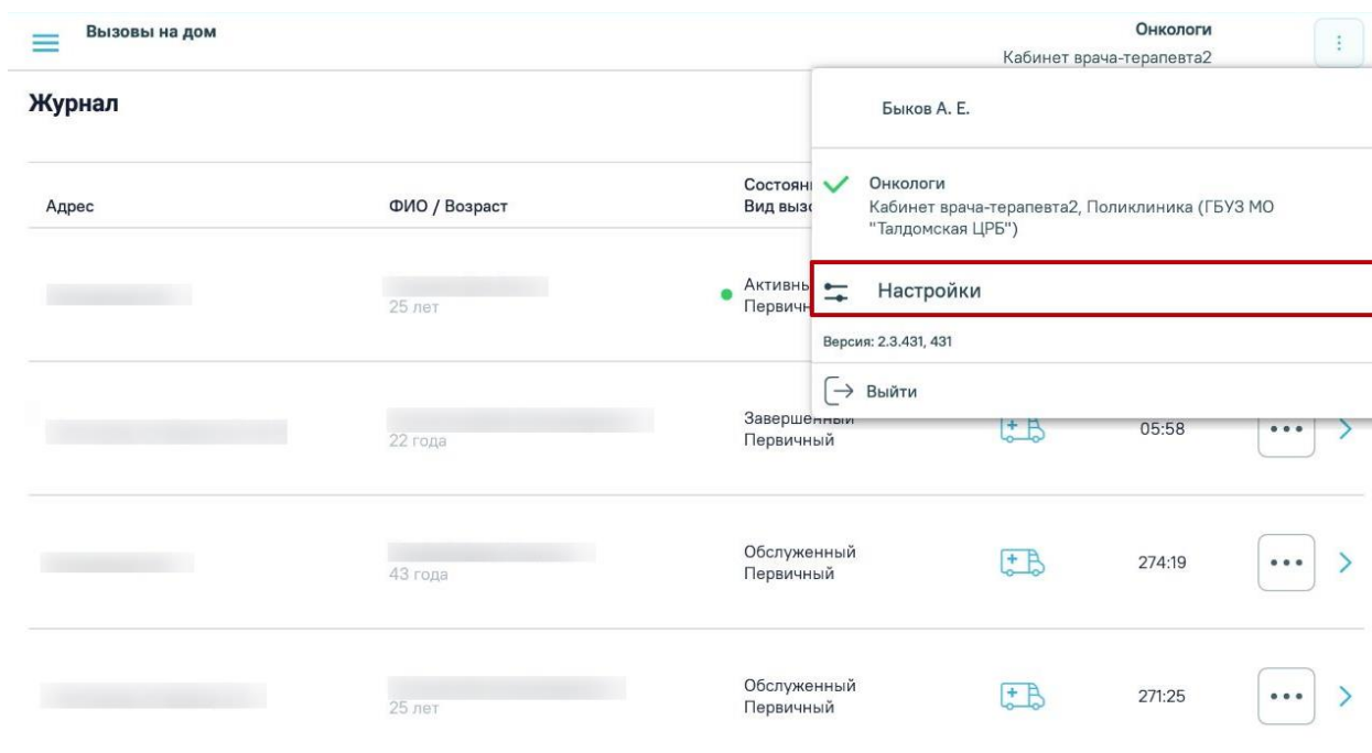
Рисунок 1329. Кнопка «Настройки»
