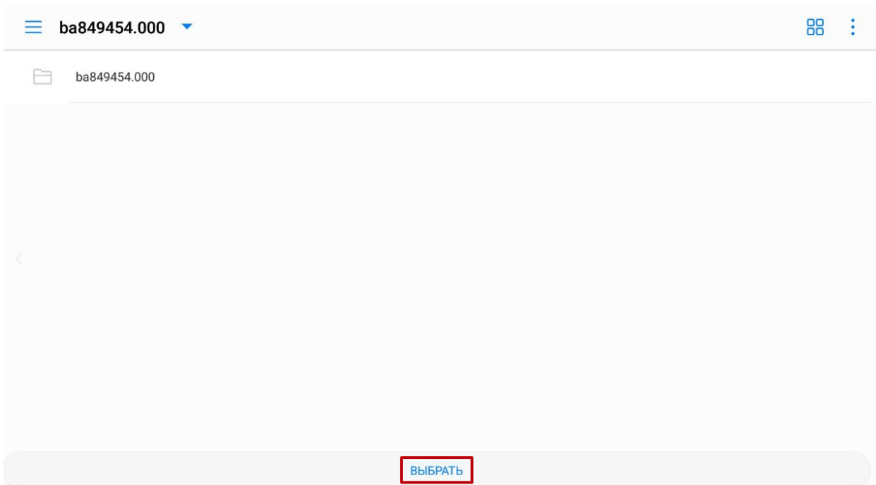
Рисунок 1333. Выбор контейнера
