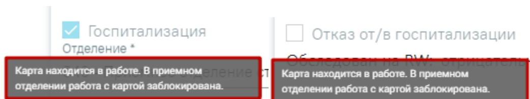
Рисунок 236. Всплывающая подсказка
