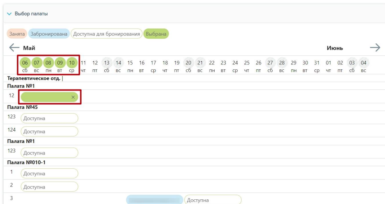
Рисунок 820. Выбор койки
