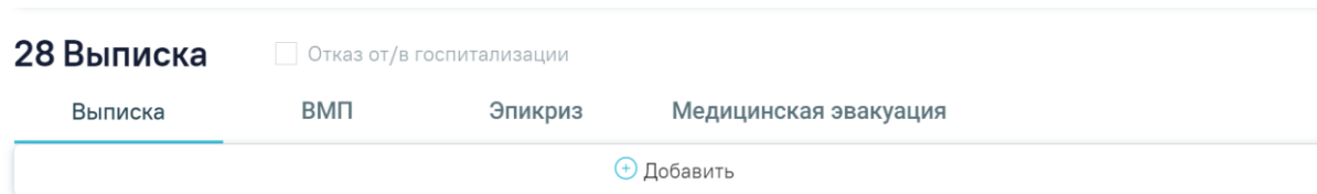
Рисунок 651. Вкладка «Выписка»
