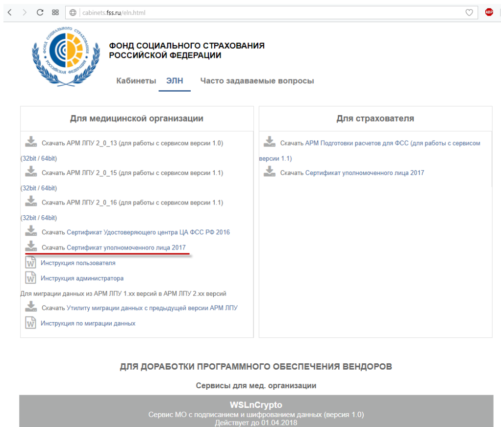
Рисунок 855. Сайт ФСС
