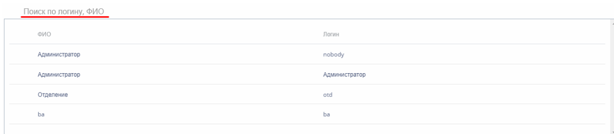
Рисунок 1017. Выбор пользователя
