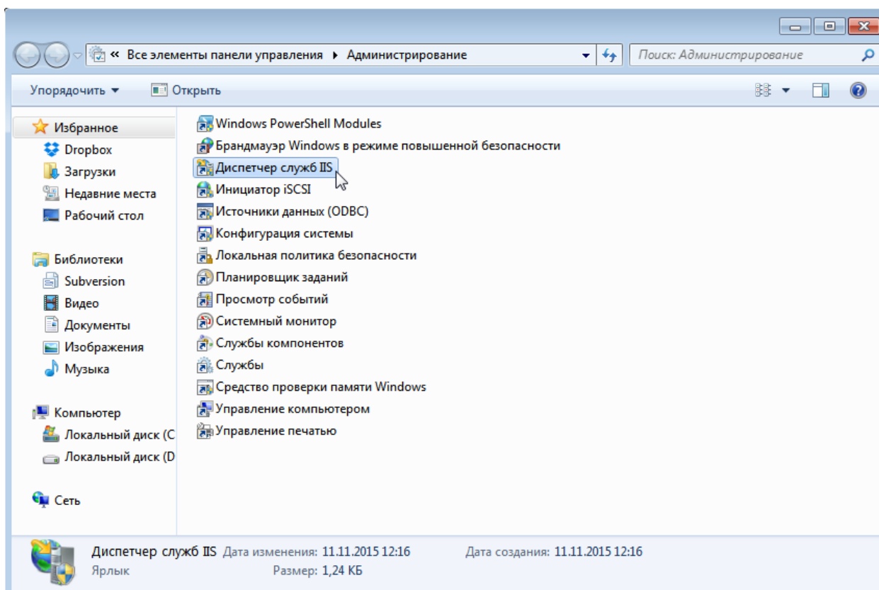
Рисунок 720. Запуск IIS
