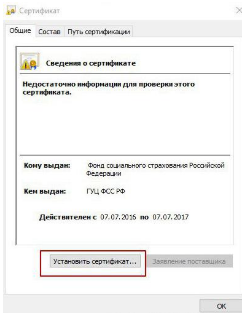
Рисунок 825. Окно «Сертификат»
