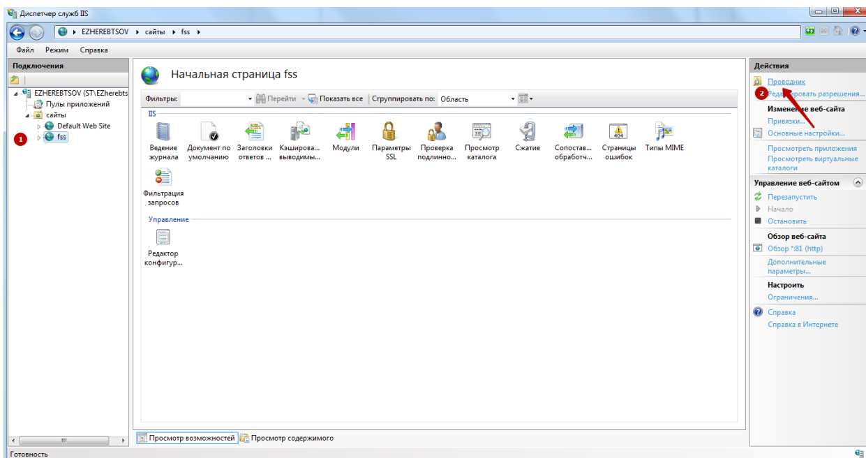
Рисунок 704. Консоль ISS
