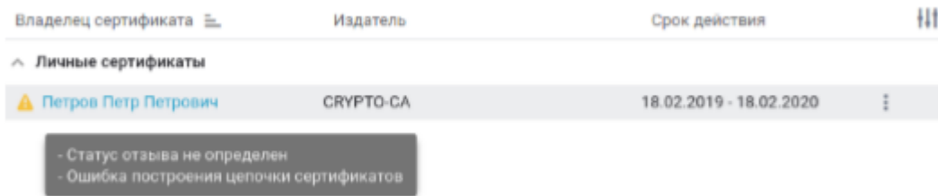
Рисунок 706. Предупреждающие сообщения
