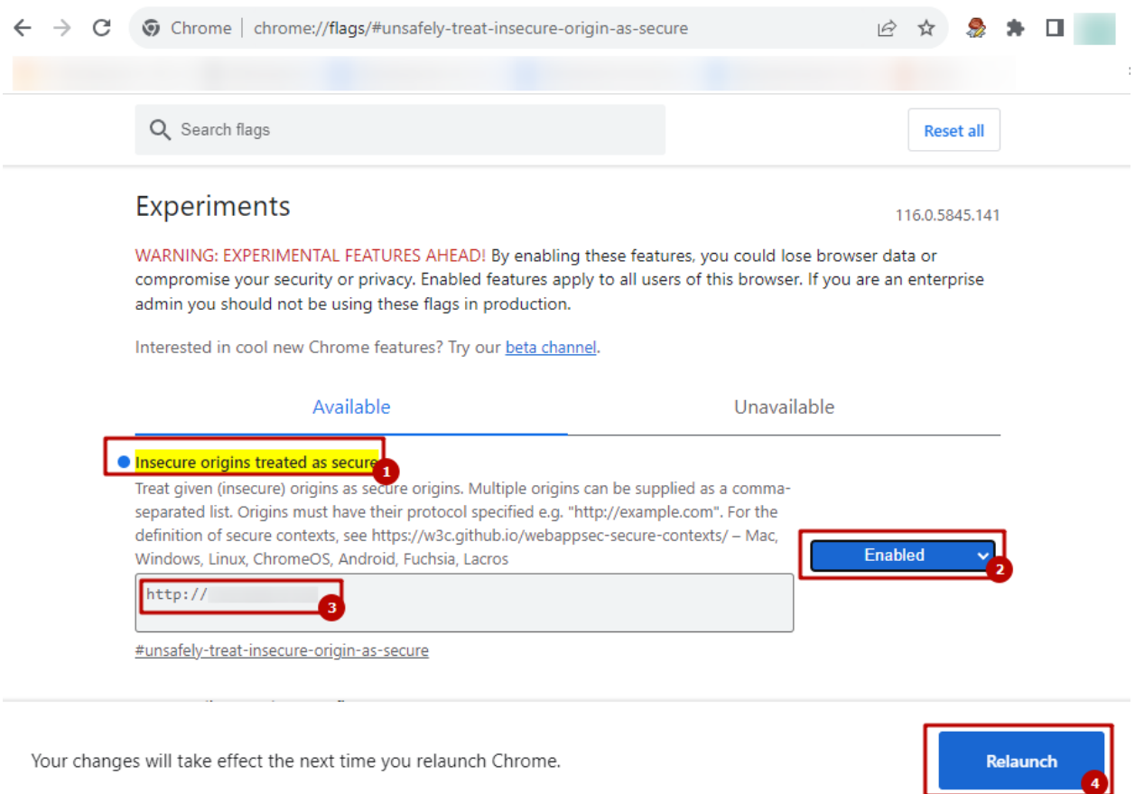
Рисунок 475. Установка флага Insecure origins treated as secure
