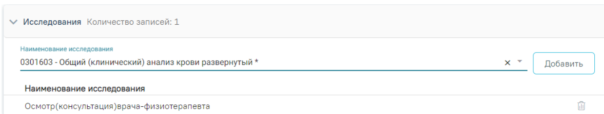
Рисунок 838. Раздел «Исследования»
