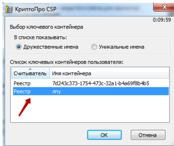
Рисунок 739. Выбор контейнера
