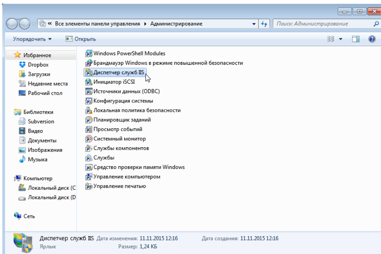
Рисунок 609. Запуск IIS
