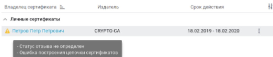
Рисунок 799. Предупреждающие сообщения
