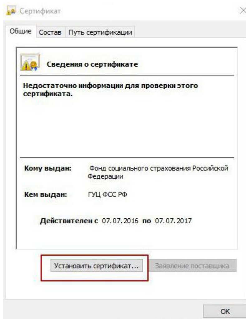
Рисунок 735. Окно «Сертификат»
