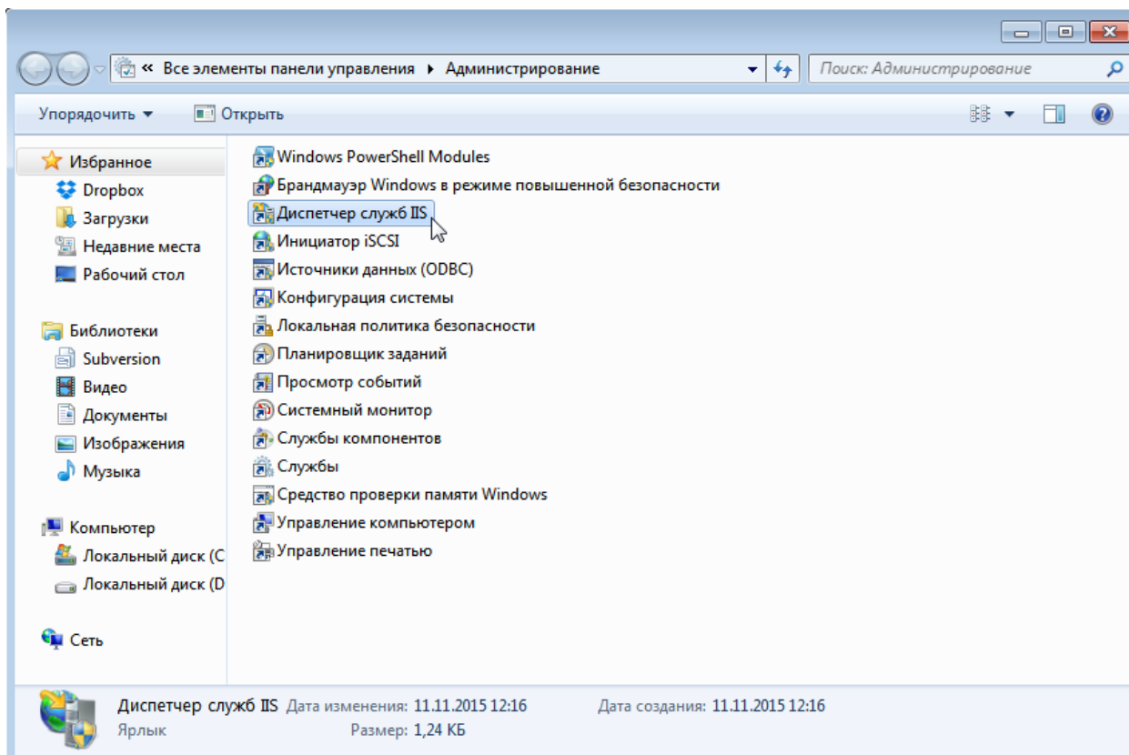
Рисунок 630. Запуск IIS
