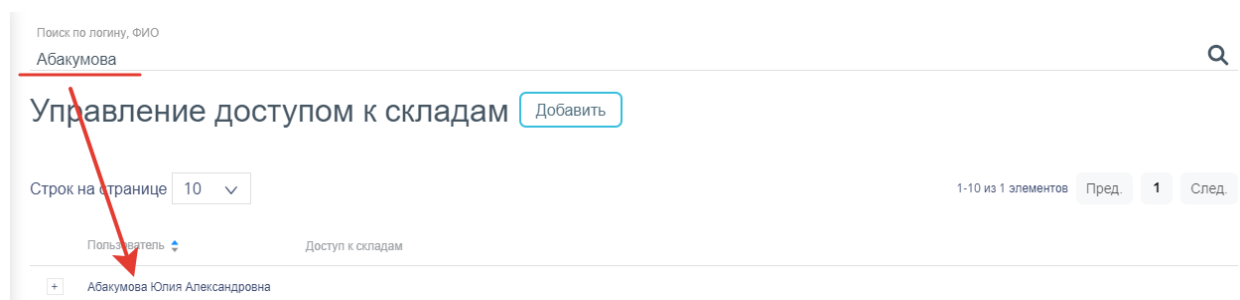
Рисунок 921. Результат поиска
