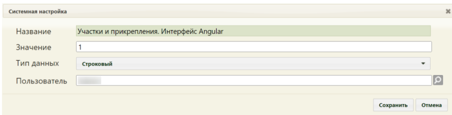
Рисунок 476. Системная настройка «Участки и приращения. Интерфейс Angular» Форма настройки закроется. Настройка будет включена.
