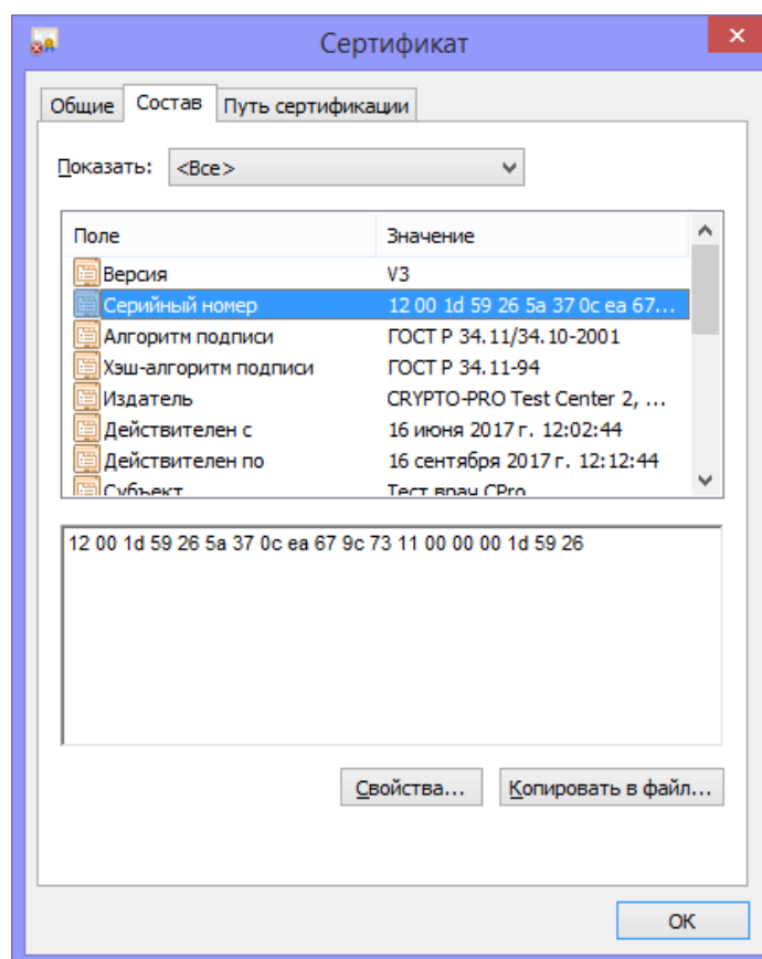
Рисунок 865. Выбор сертификата при подписании ЭП
