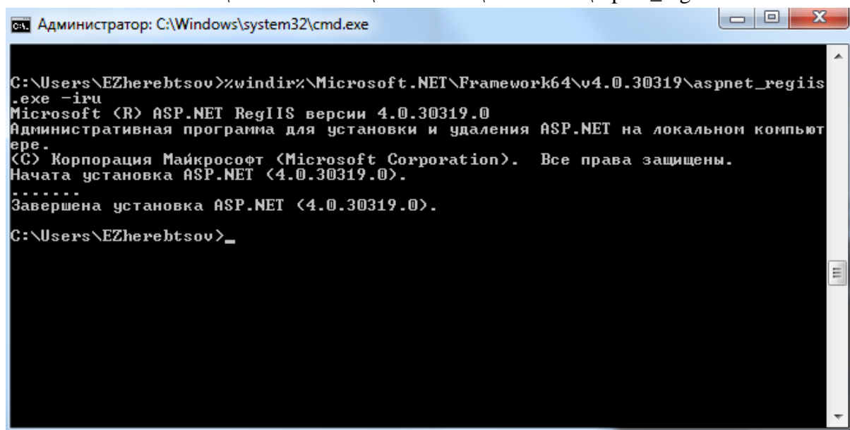
Рисунок 834. Команда регистрации ASP.NET в консоли
