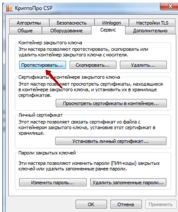
Рисунок 806. Окно «КриптоПро CSP», вкладка «Сервис»
