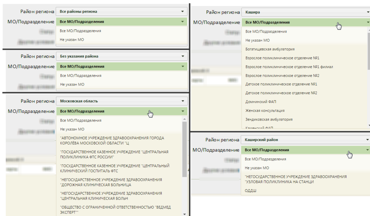
Рисунок 5. Выбор МО/подразделения
