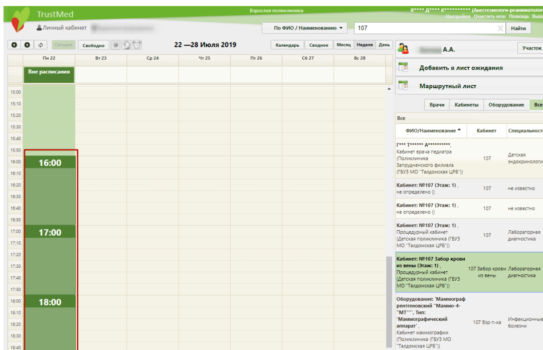
Рисунок 28. Расписание кабинета
