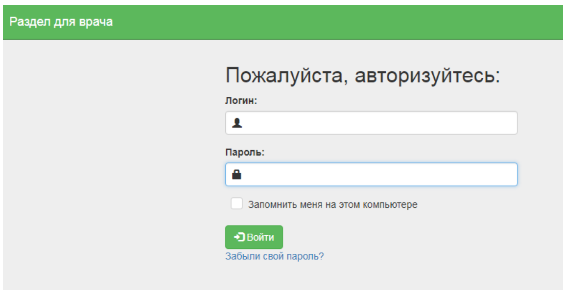
Рисунок 35. Окно авторизации
