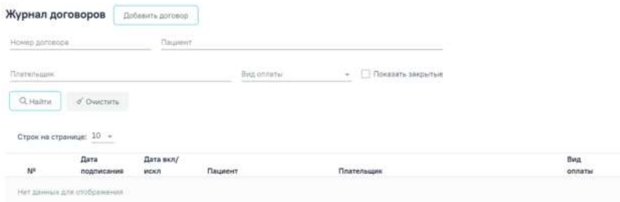
Рисунок 35. Журнал договоров
