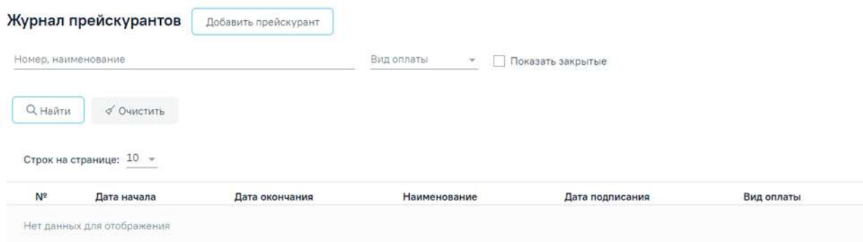
Рисунок 14. Журнал прейскурантов
