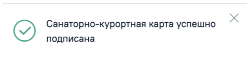
Рисунок 27. Информационное сообщение
