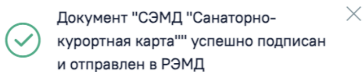
Рисунок 39. Информационное сообщение
