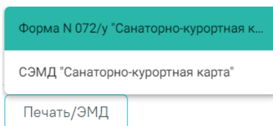
Рисунок 36. Кнопка «Печать/ЭМД»
