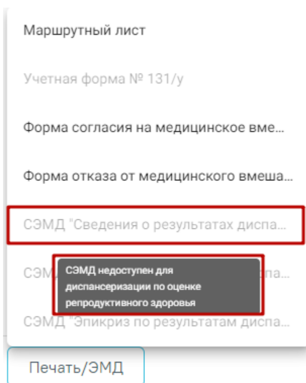
Рисунок 999. Всплывающая подсказка
