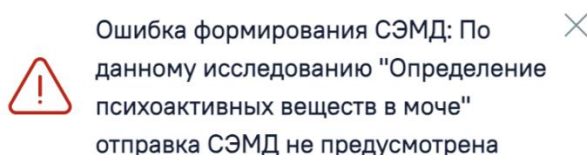
Рисунок 1037. Предупреждающее сообщение
