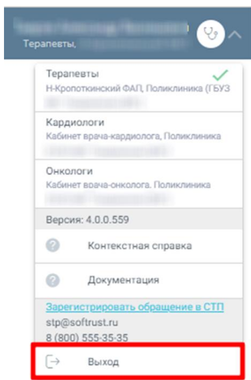
Рисунок 1129. Закрытие журнала
