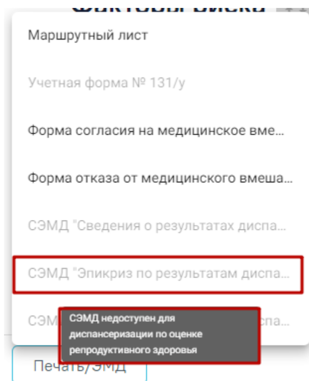
Рисунок 1033. Всплывающая подсказка
