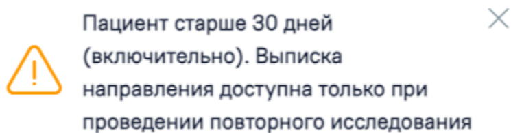
Рисунок 736. Предупреждающее сообщение
