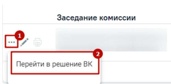
Рисунок 610. Дополнительные действия
