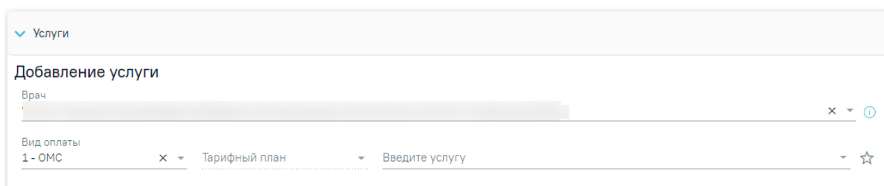
Рисунок 476. Блок «Услуги»
