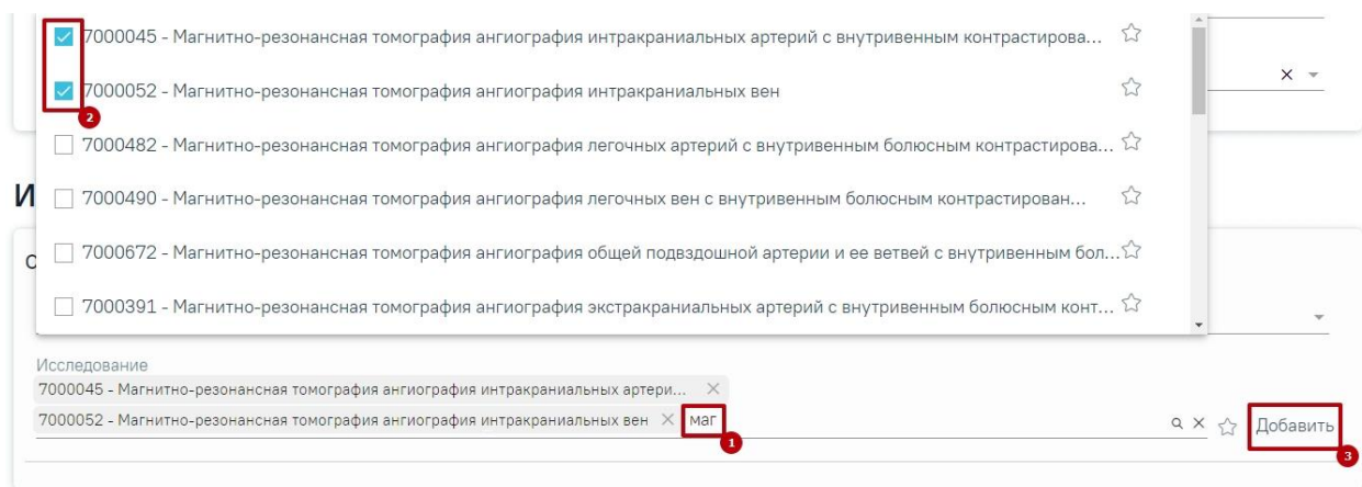
Рисунок 269. Добавление исследования
