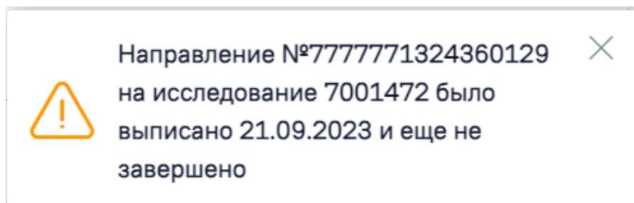
Рисунок 272. Предупреждающее сообщение
