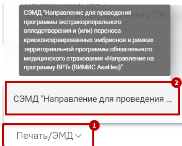
Рисунок 768. Кнопка «Печать/ЭМД»
