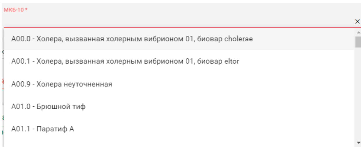
Рисунок 285. Список диагнозов
