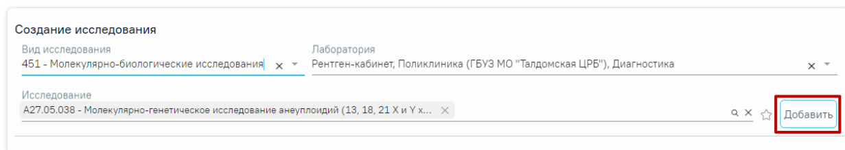
Рисунок 426. Добавление исследования
