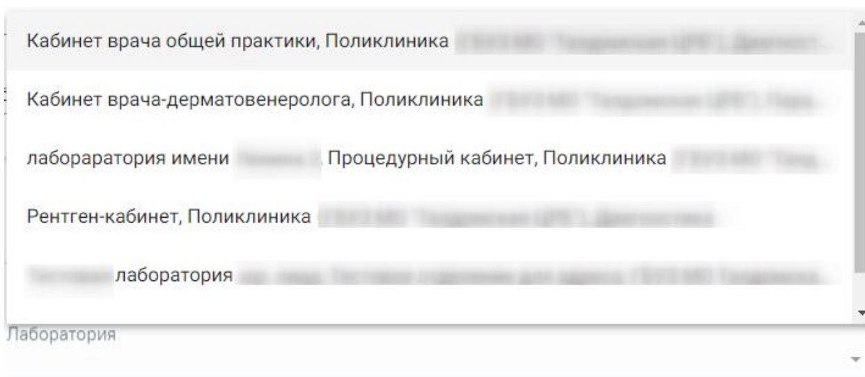
Рисунок 293. Выбор лаборатории
