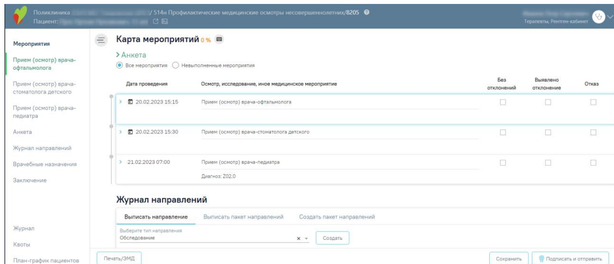
Рисунок 98. Заголовок «Анкета»
