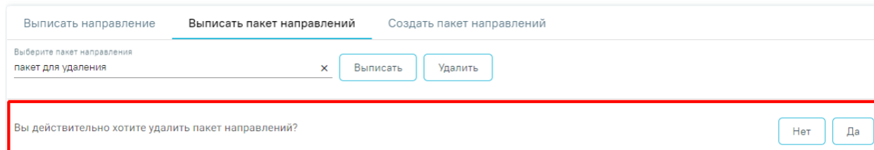
Рисунок 197. Подтверждение действия
