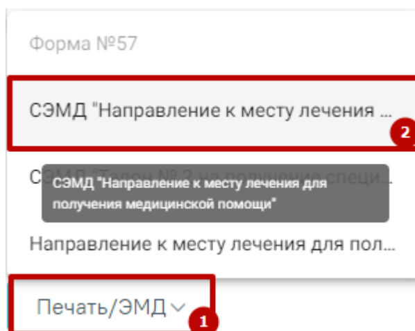
Рисунок 406. Кнопка «Печать/ЭМД»
