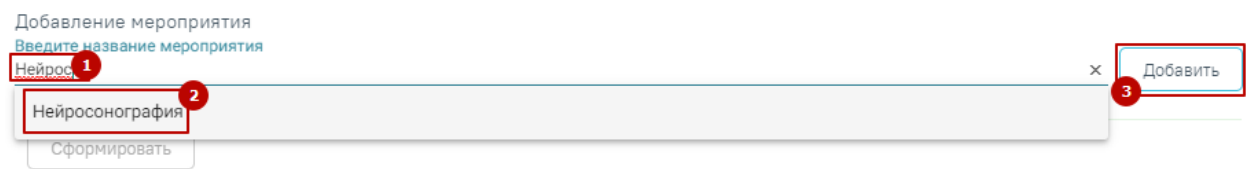
Рисунок 488. Выбор мероприятия
