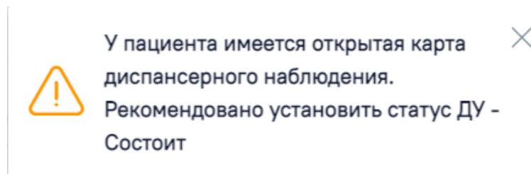
Рисунок 160. Предупреждающее сообщение
