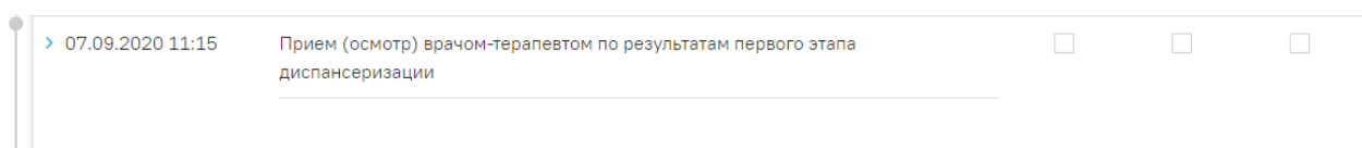
Рисунок 118. Выбор мероприятия
