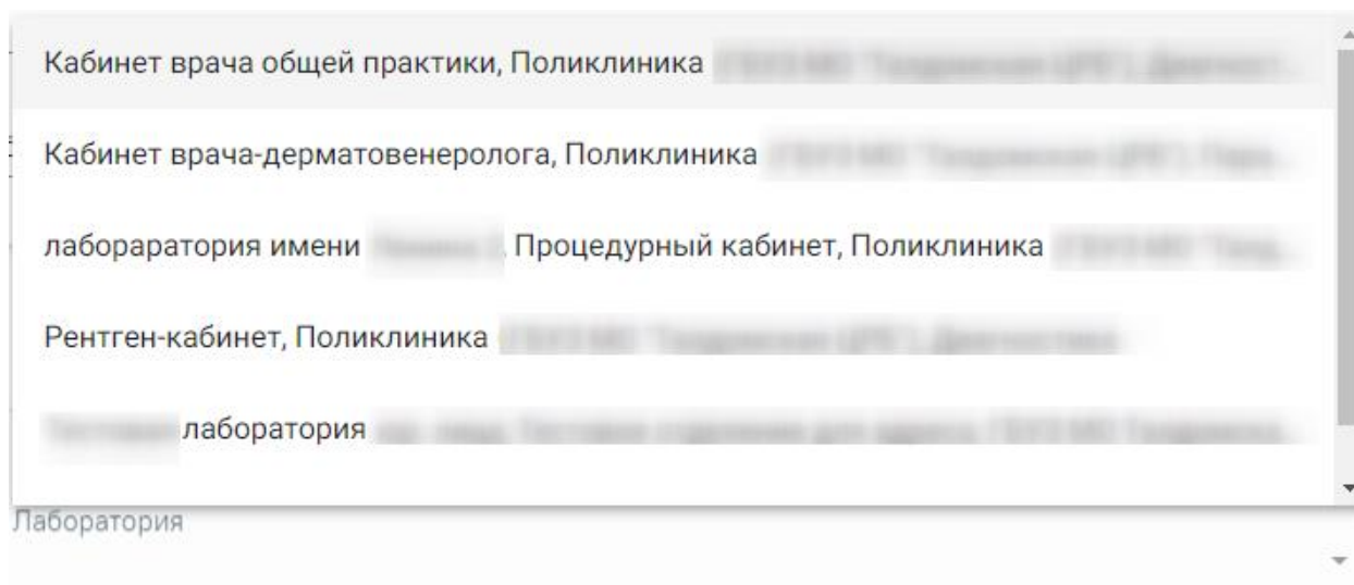
Рисунок 312. Выбор лаборатории
