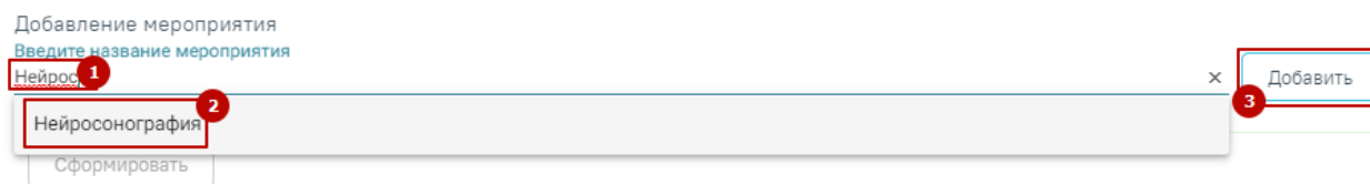
Рисунок 512. Выбор мероприятия
