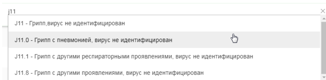
Рисунок 126. Ввод диагноза
