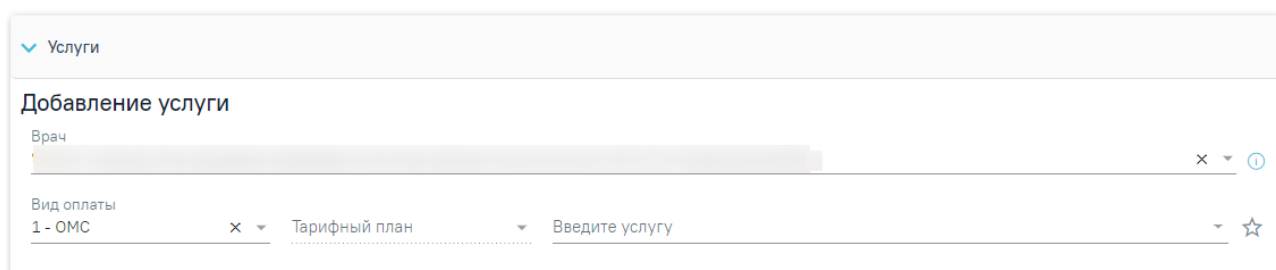
Рисунок 359. Блок «Услуги»
