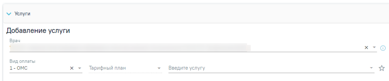
Рисунок 253. Блок «Услуги»
