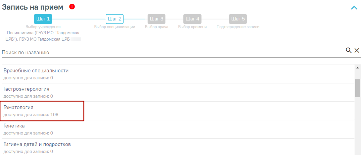
Рисунок 503. Выбор специализации
