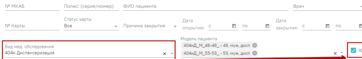
Рисунок 617. Флажок «УД»
