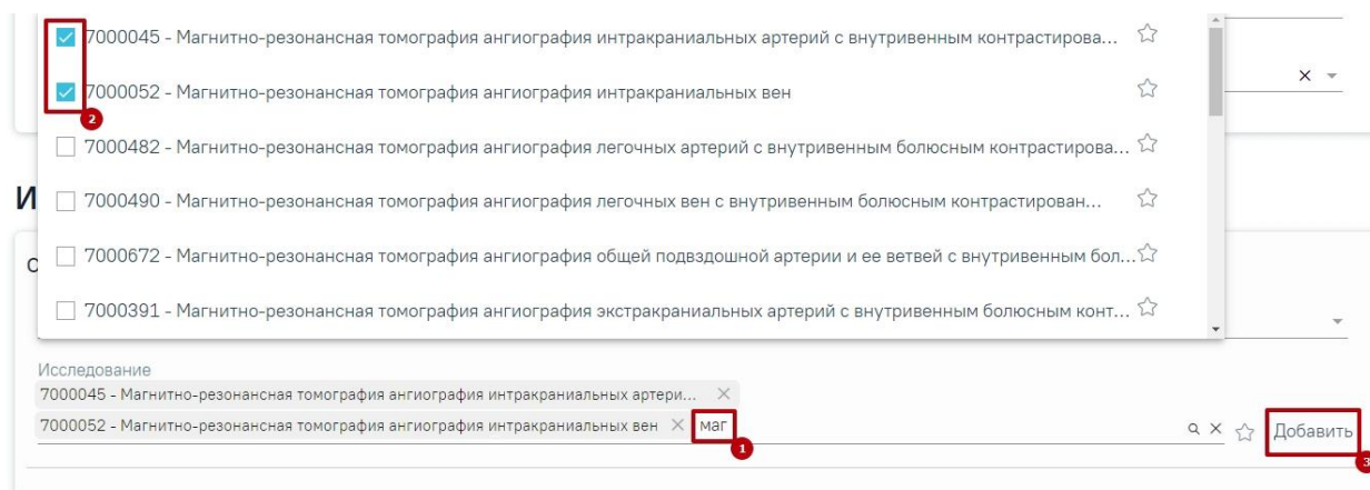
Рисунок 219. Добавление исследования
