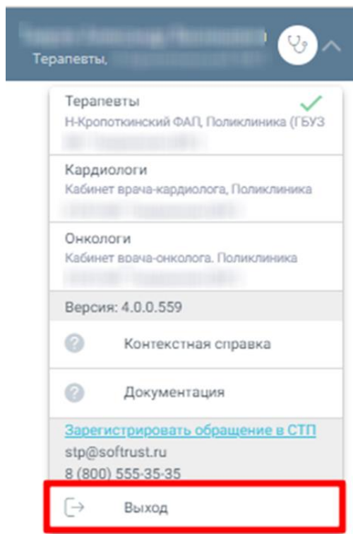
Рисунок 630. Закрытие журнала
