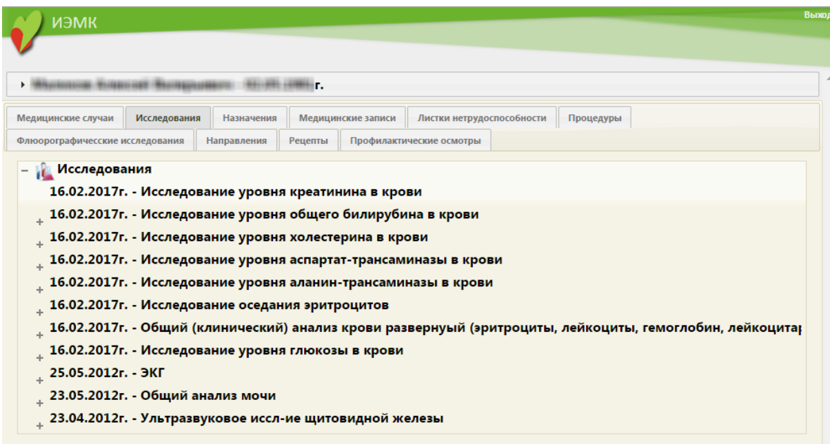
Рисунок 442. Вкладка «Исследования»
