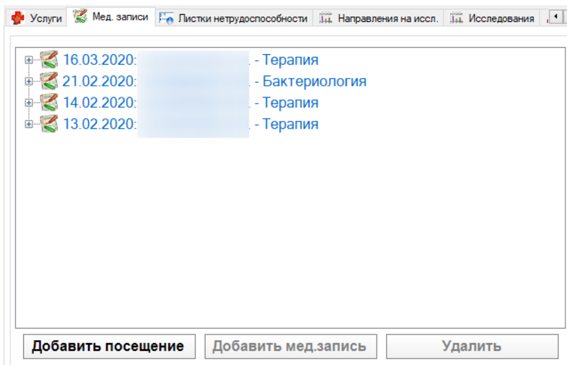
Рисунок 373. Вкладка «Посещения»
