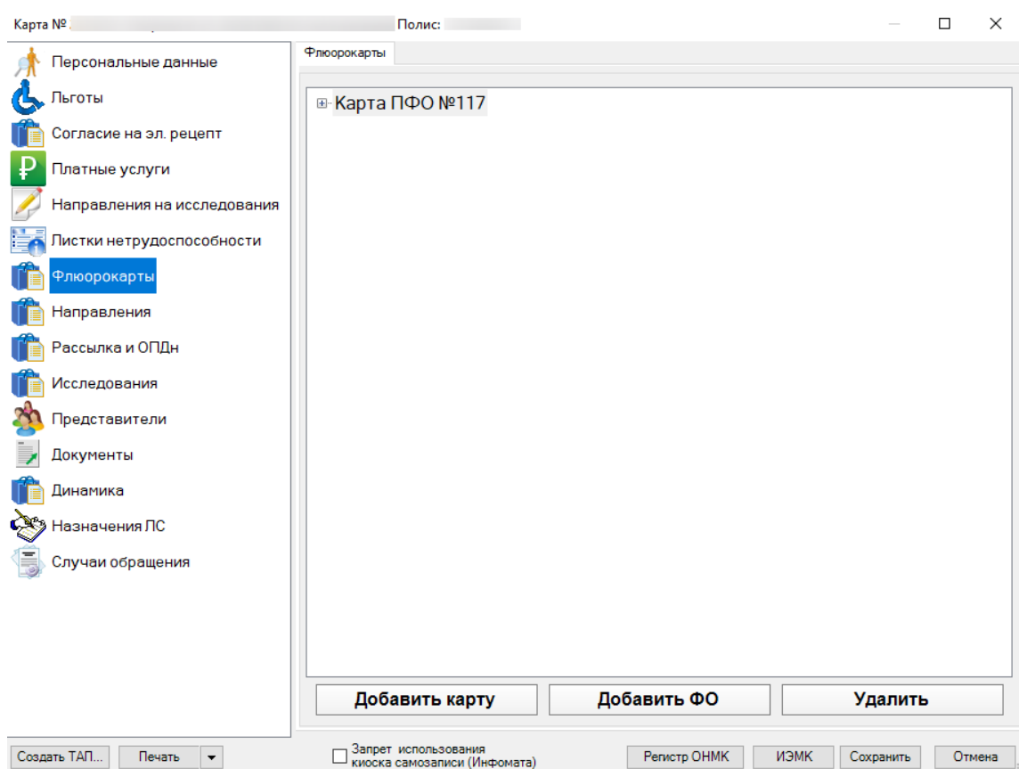
Рисунок 295. Вкладка «Флюорокарты»
