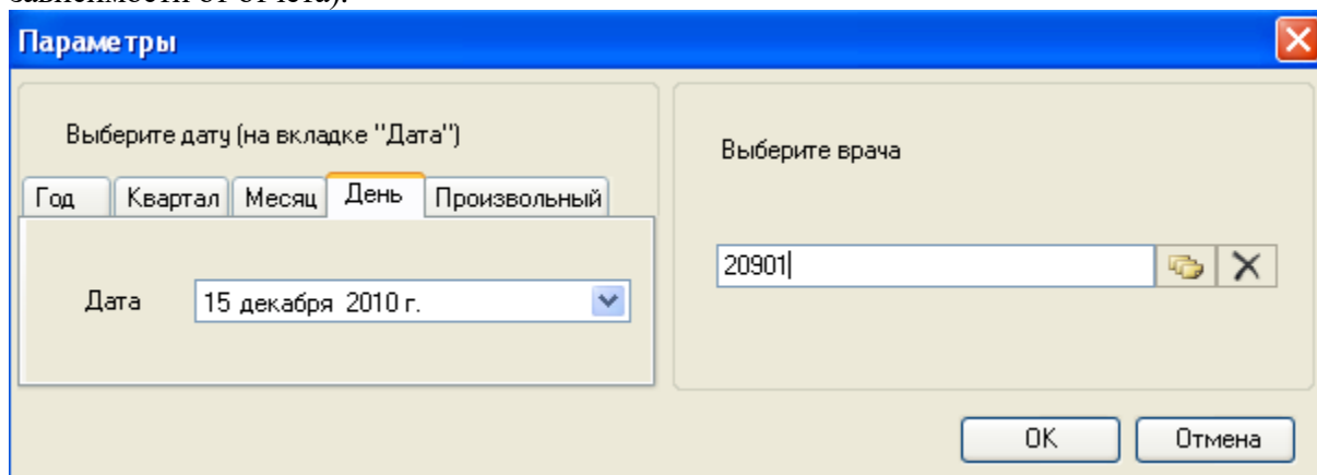
Рисунок 1231. Окно «Параметры»
