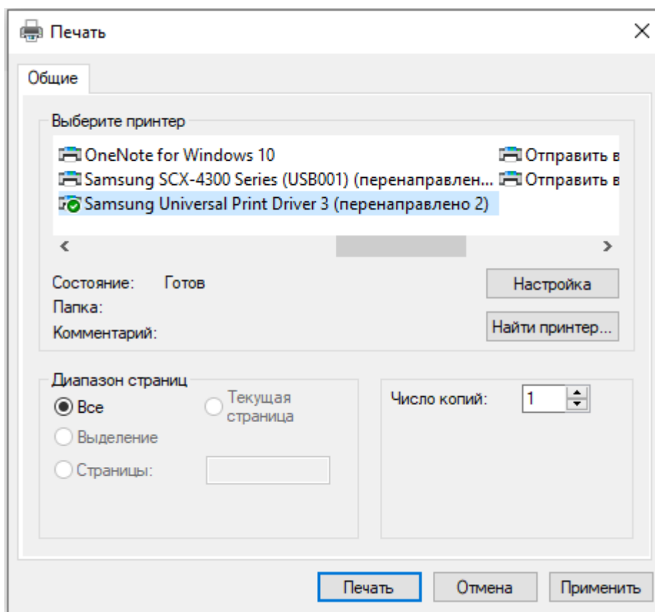
Рисунок 394. Печать осмотра
