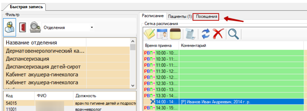
Рисунок 210. Вкладка «Посещения»
