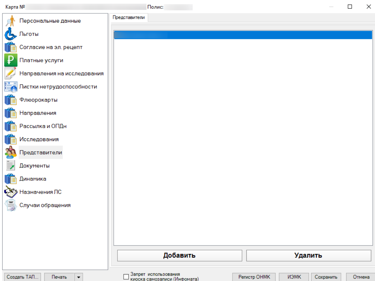
Рисунок 308. Вкладка «Представители»
