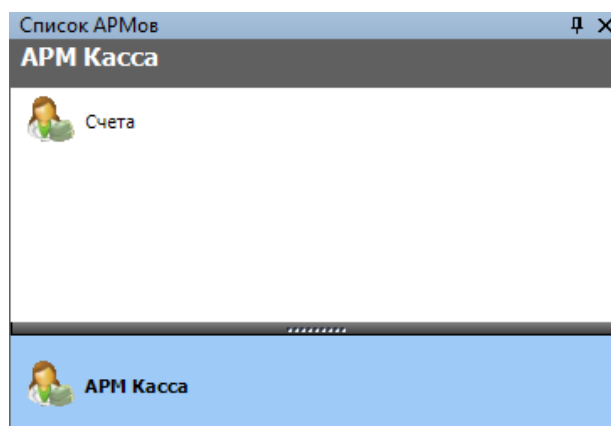
Рисунок 1172. АРМ «Касса»
