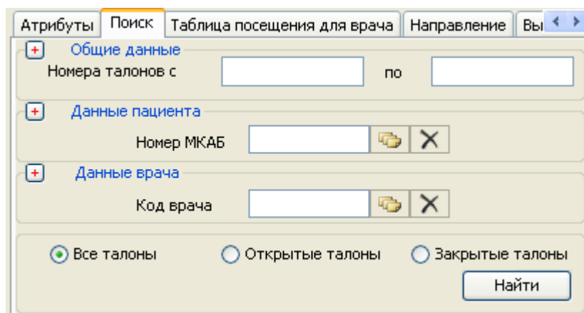
Рисунок 718. Вкладка «Поиск»
