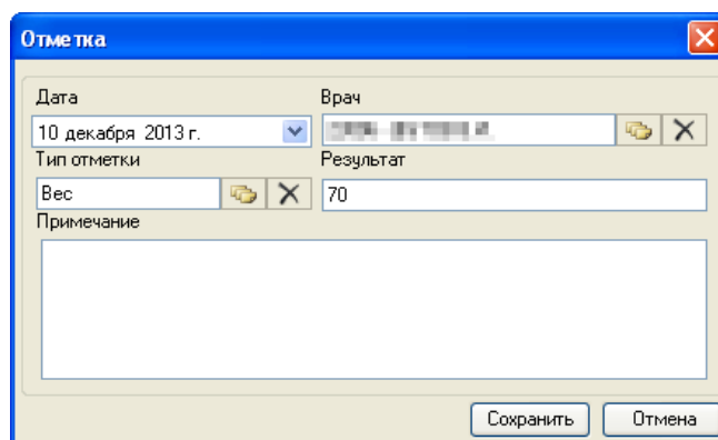
Рисунок 988. Окно «Отметка»
