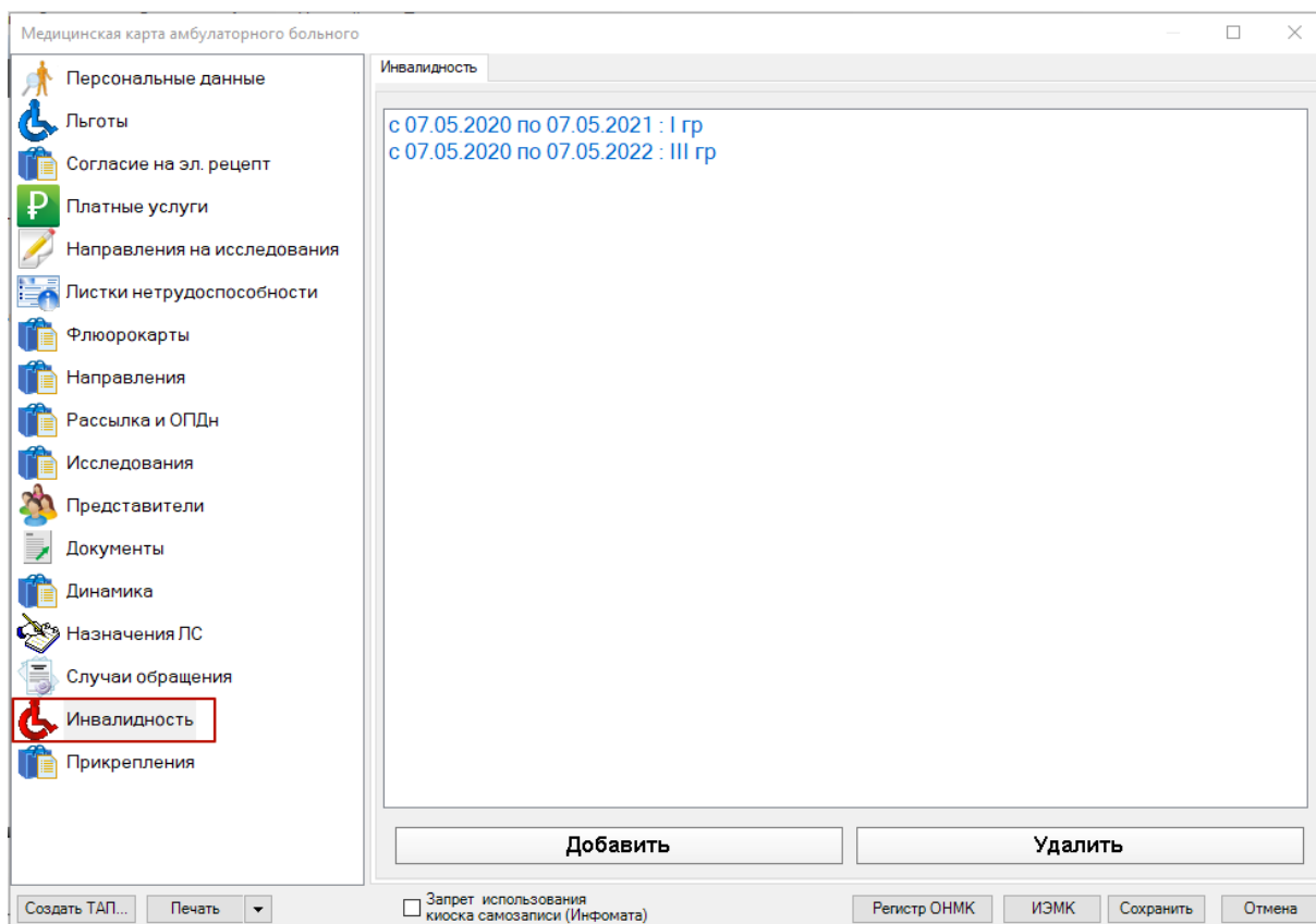
Рисунок 317. Вкладка «Инвалидность»
