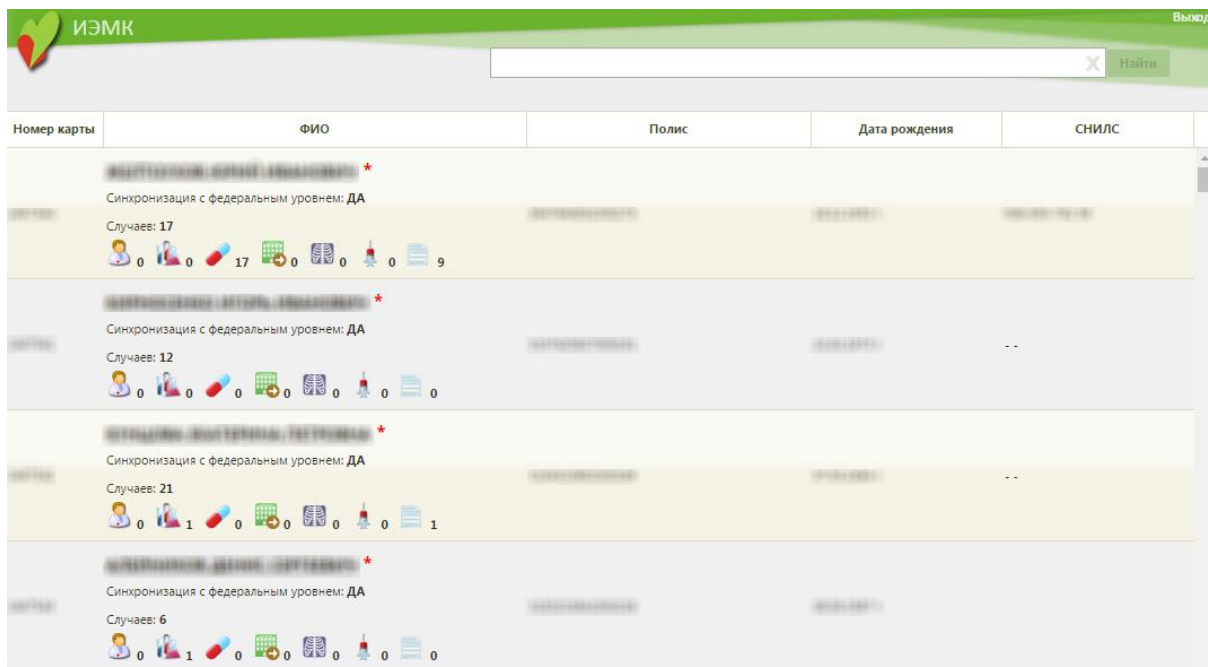
Рисунок 437. Список ИЭМК
