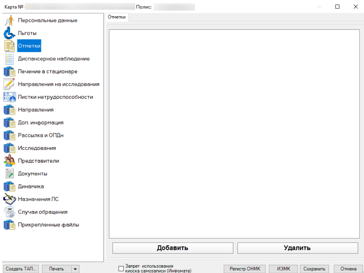
Рисунок 324. Отметки пациента
