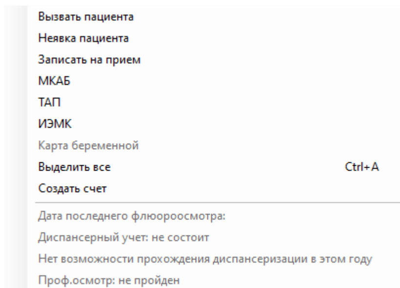
Рисунок 244. Контекстное меню
