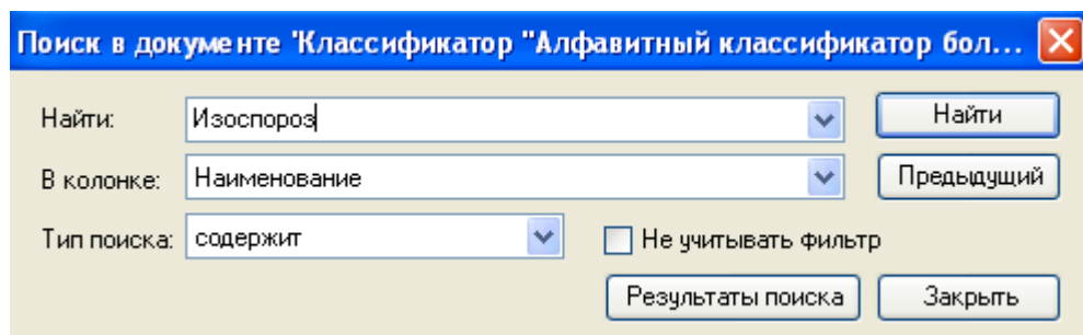
Рисунок 14. Маркер на найденной записи
