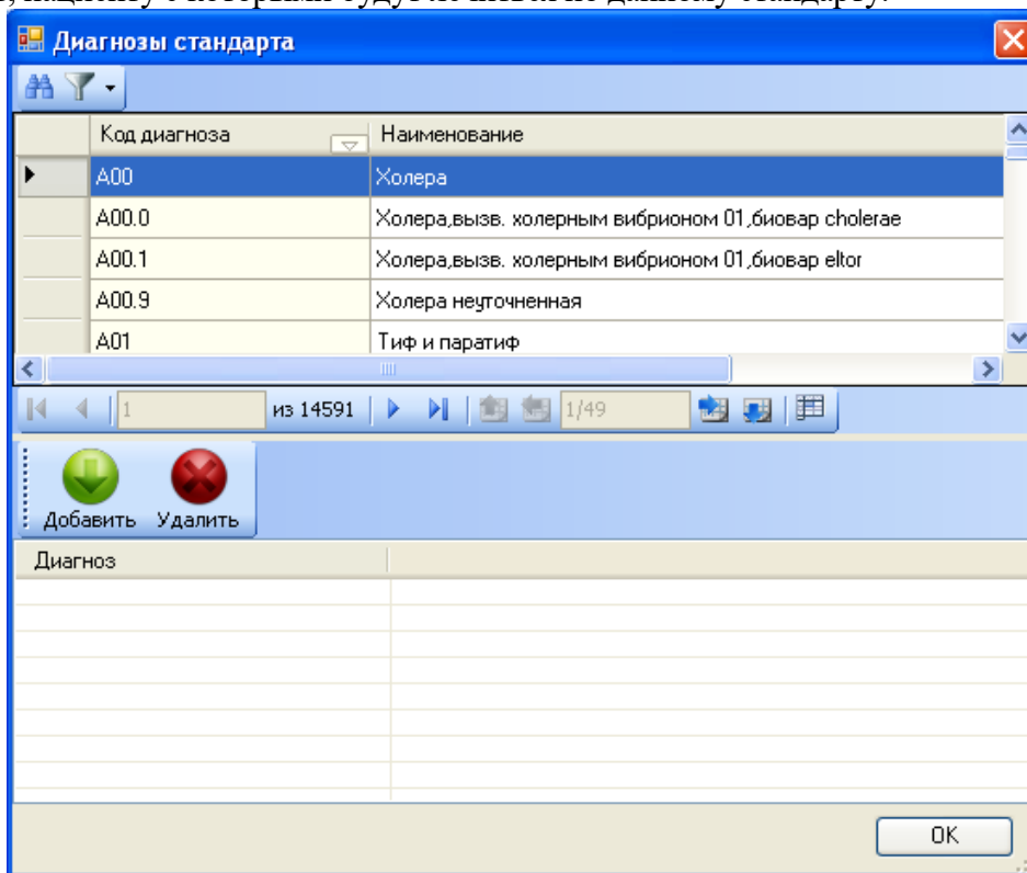
Рисунок 139. Окно «Диагнозы стандарта»
