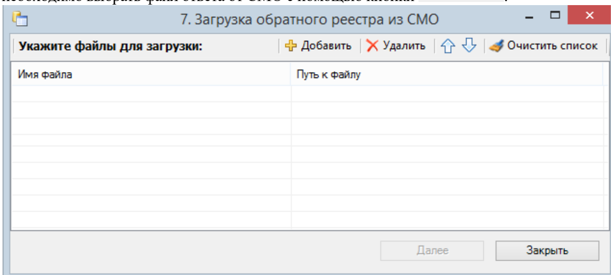
Рисунок 674. Окно загрузки обратного реестра из СМО
