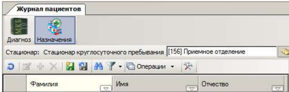
Рисунок 381. Кнопка «Назначение»
