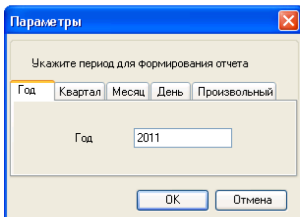
Рисунок 331. Окно «Параметры»
