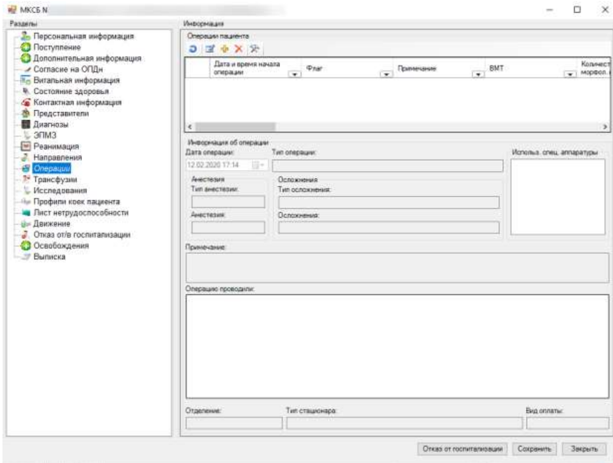
Рисунок 140. Окно «Операции»
