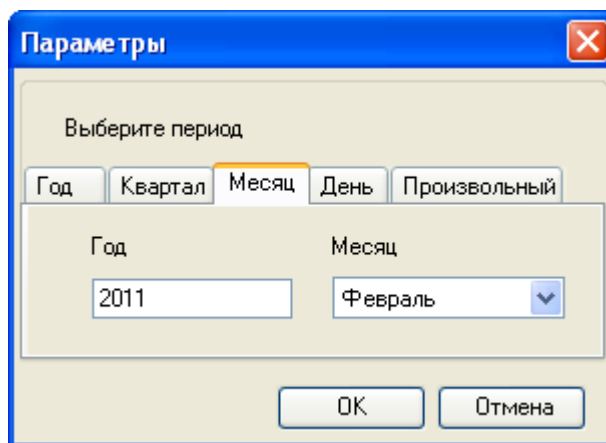
Рисунок 466. Окно «Параметры»
