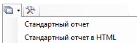
Рисунок 468. Кнопки «Отчеты»
