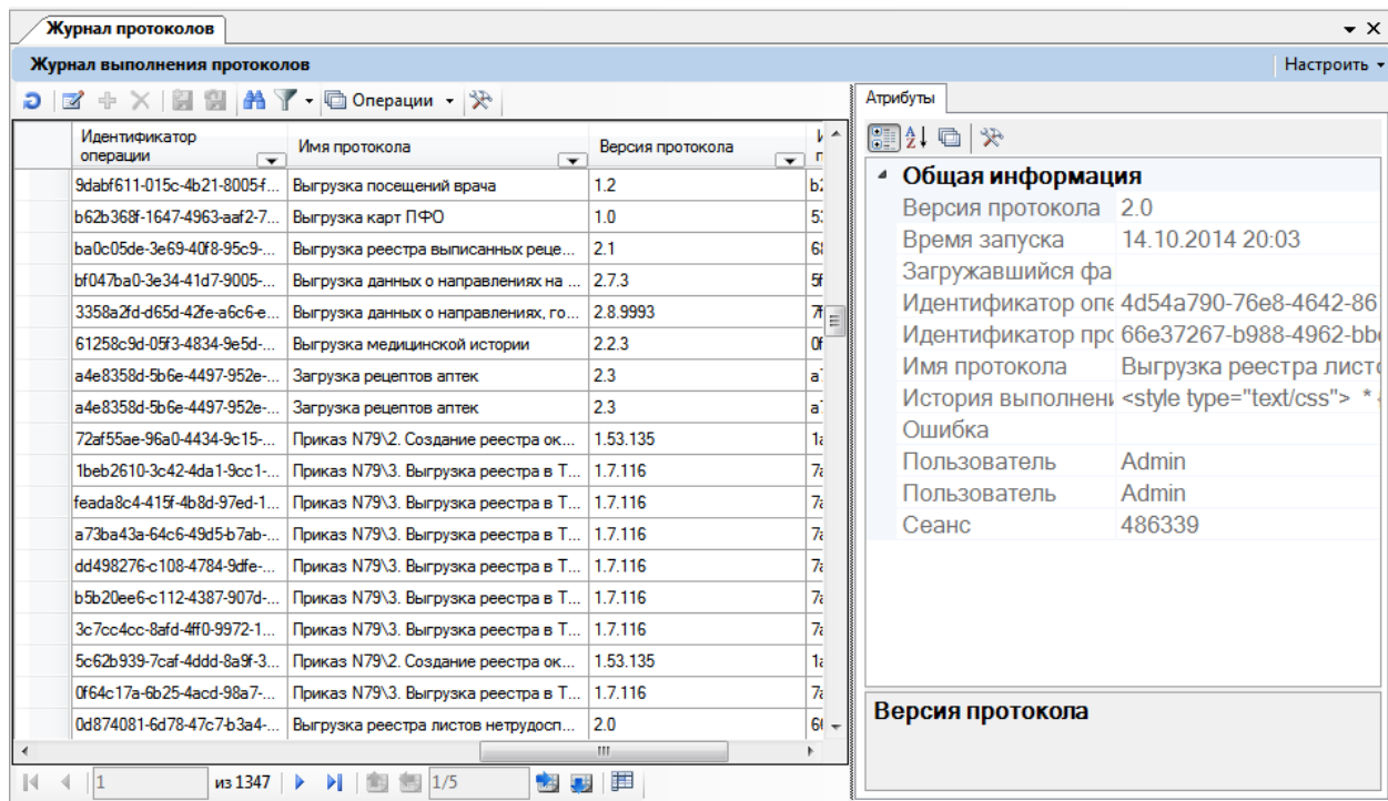
Рисунок 84. Журнал протоколов
