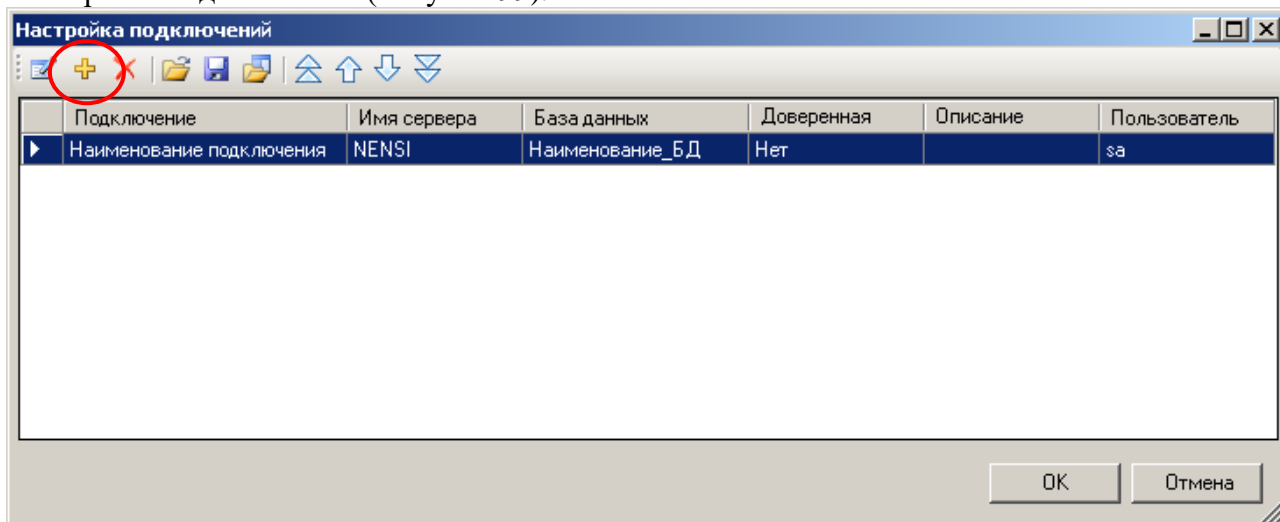
Рисунок 98. Редактирование подключений
