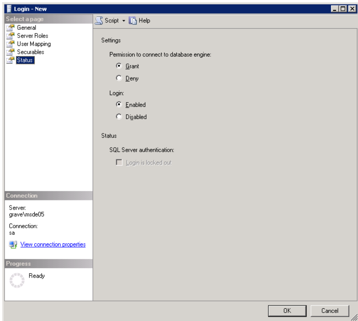
Рисунок 107. Вкладка «Status»
