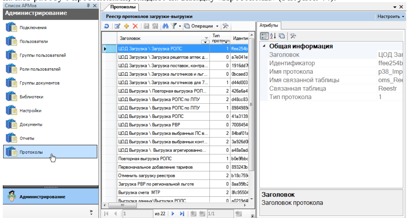
Рисунок 44. Вкладка «Протоколы»
