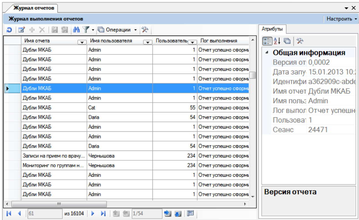
Рисунок 86. Журнал отчетов
