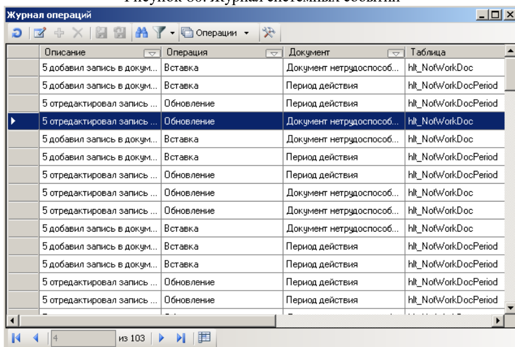
Рисунок 81. Журнал операций
