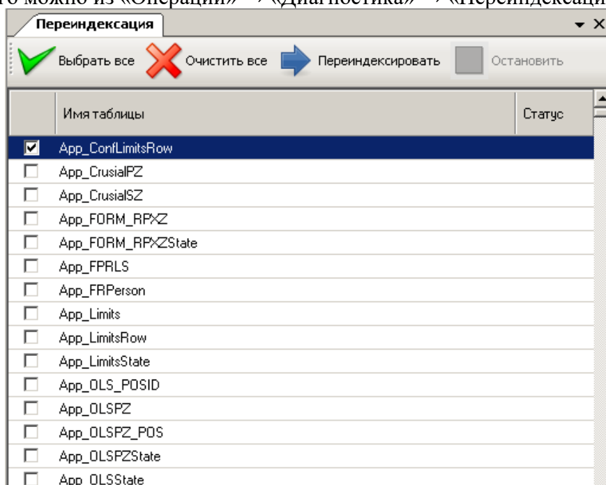
Рисунок 71. Диалог «Переиндексация»
