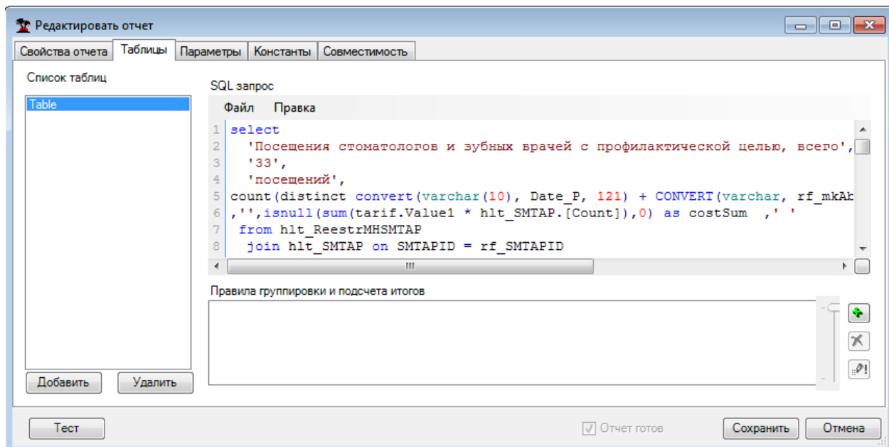
Рисунок 141. Вкладка «Таблицы»
