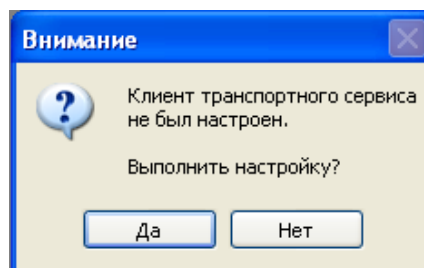
Рисунок 48. Окно «Внимание»
