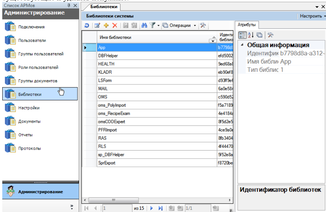
Рисунок 23. Вкладка «Библиотеки»
