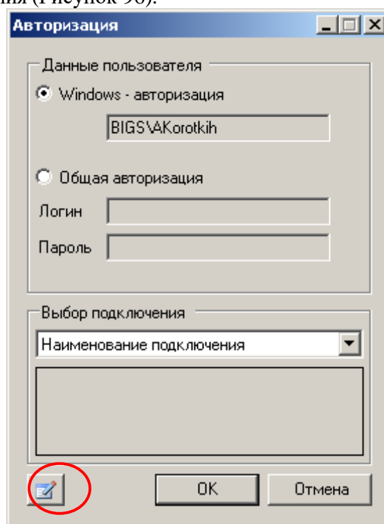
Рисунок 96. Авторизация
