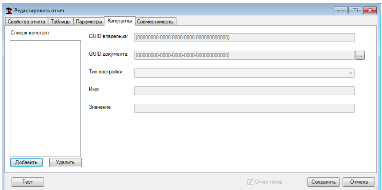
Рисунок 140. Описание констант
