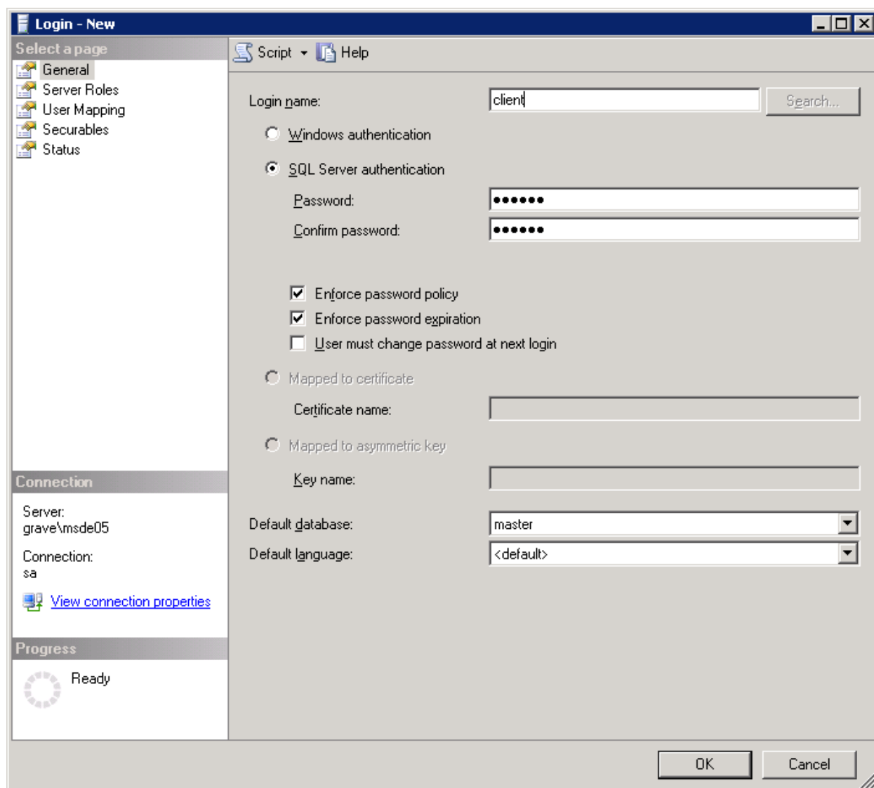
Рисунок 105. Вкладка «General»
