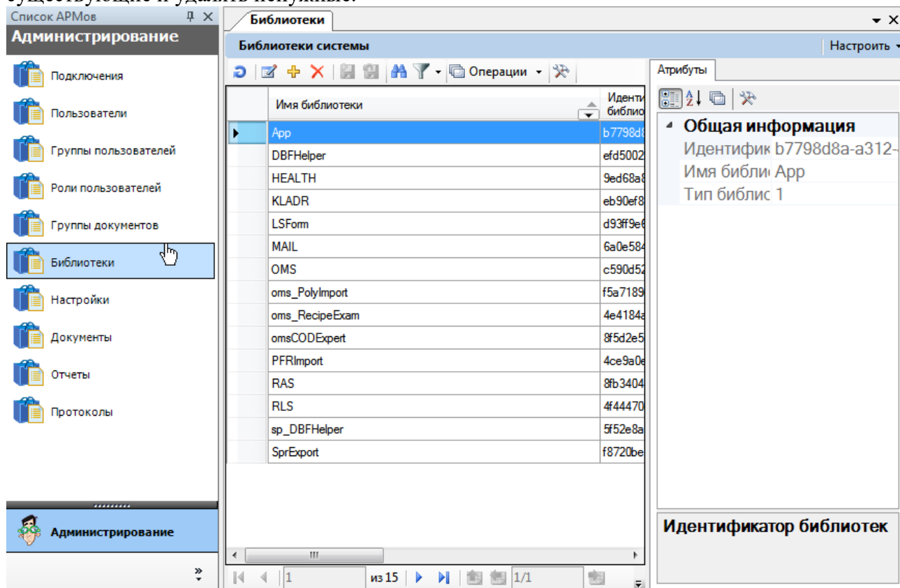
Рисунок 23. Вкладка «Библиотеки»
