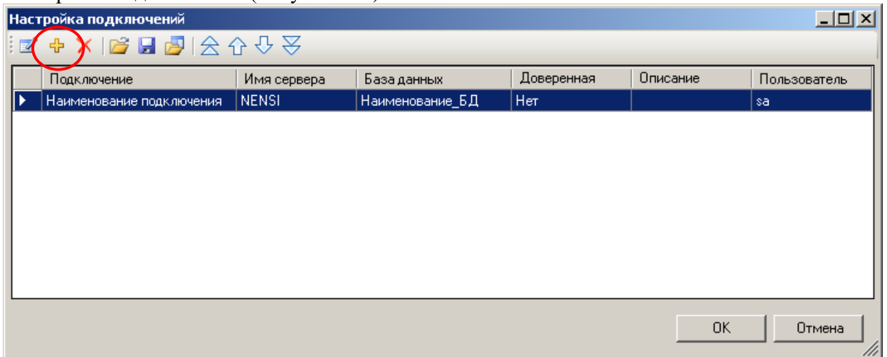
Рисунок 99. Редактирование подключений
