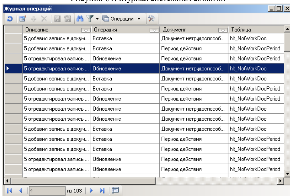
Рисунок 82. Журнал операций
