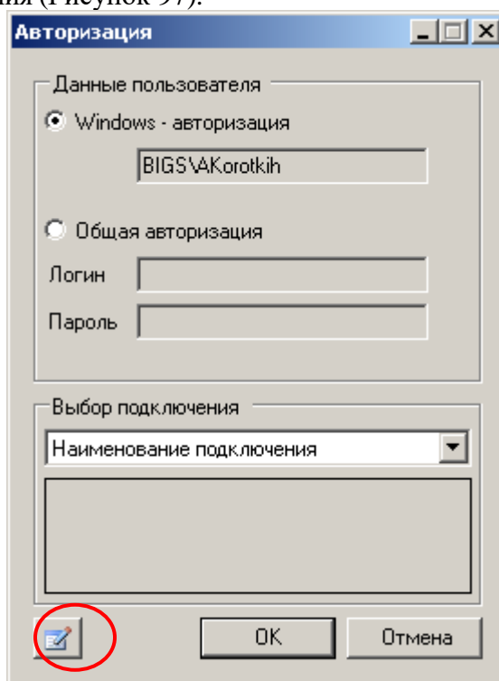
Рисунок 97. Авторизация
