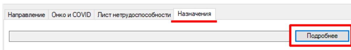
Рисунок 12. Вкладка «Назначения»
