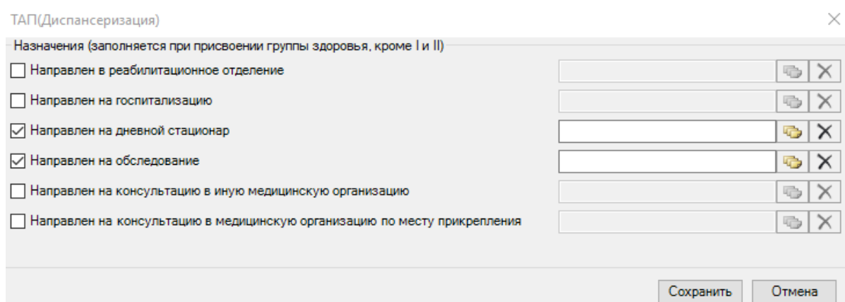
Рисунок 13. Выбор назначения
