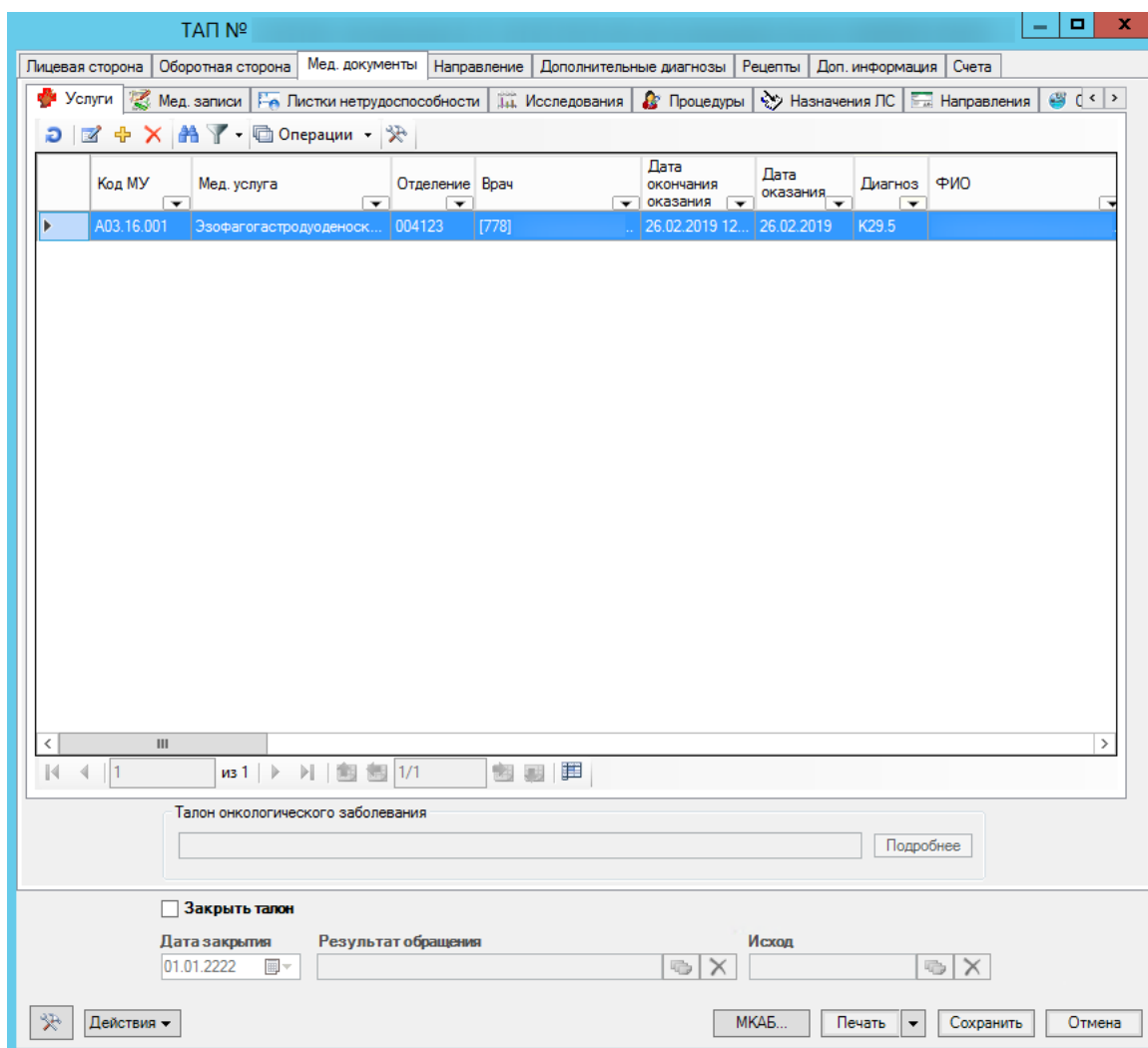
Рисунок 3. Оформление направления
