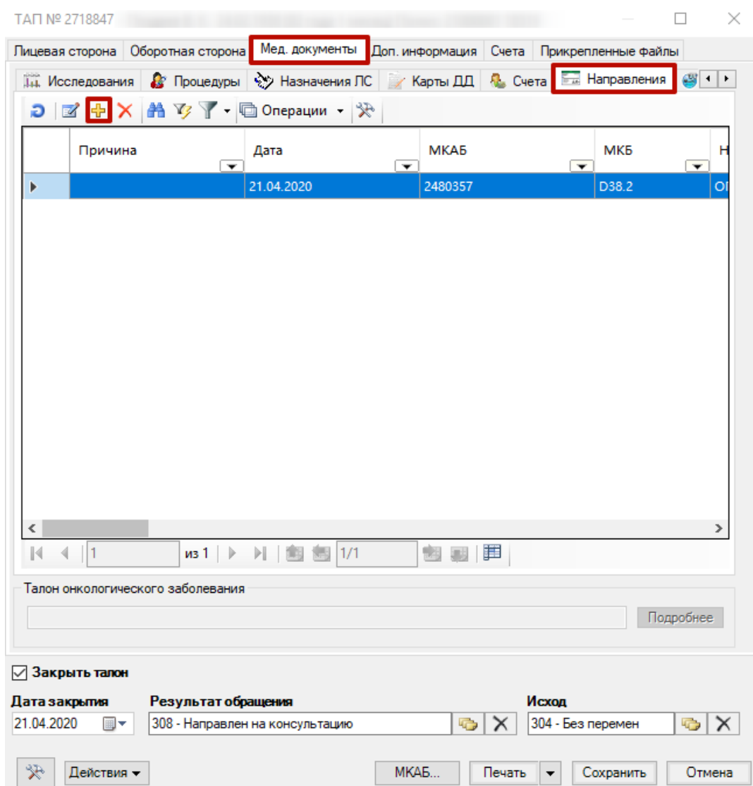
Рисунок 7. Добавление направления
