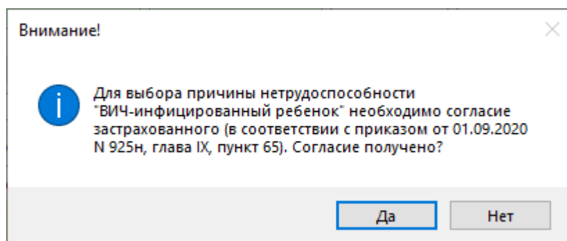
Рисунок 50. Предупреждающее сообщение
